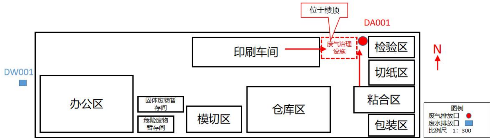
附图3 项目车间布置平面图
