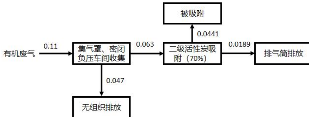
图 4-1 项目有机废气平衡图 (t/a)
