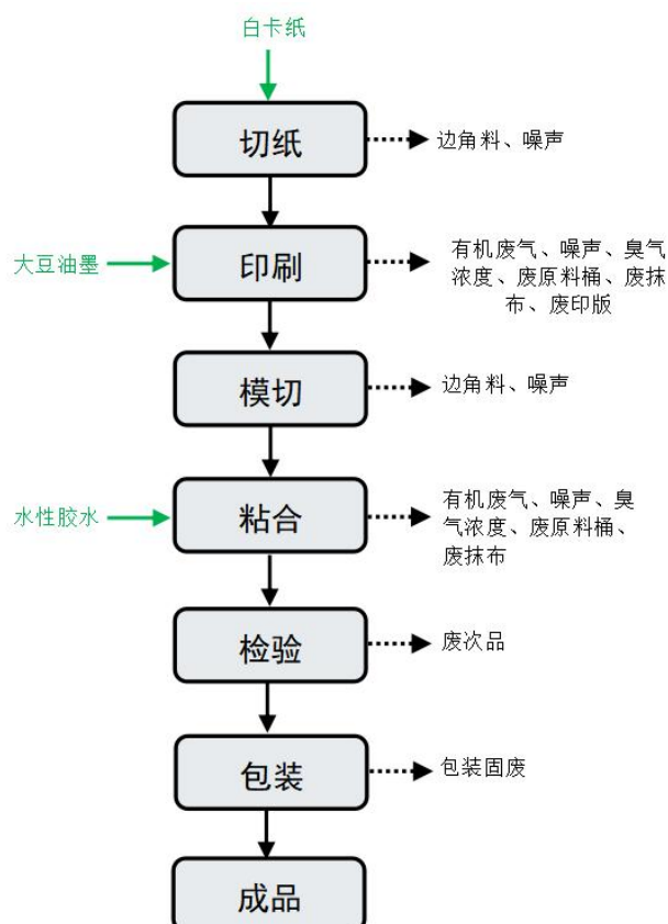
图 2-2 化妆品彩盒生产工艺流程及产污环节图
