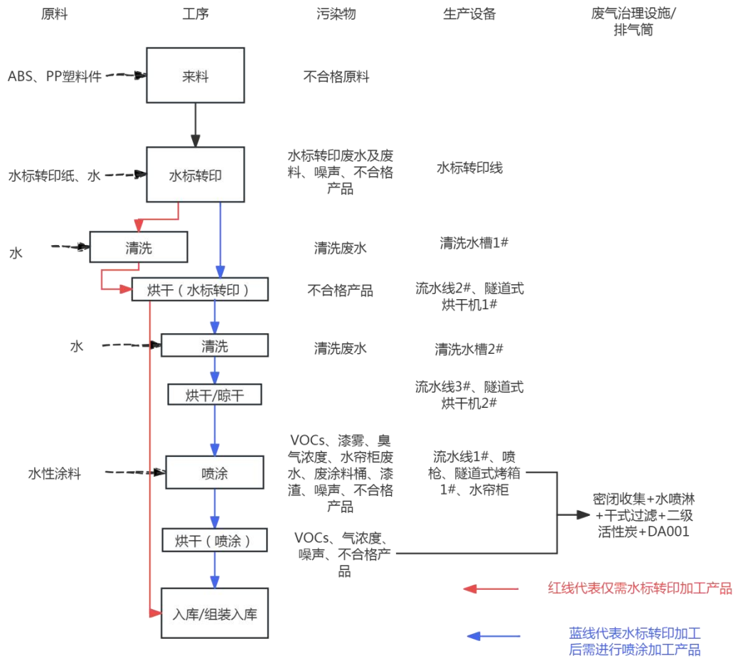
图 2-3 水标转印及喷涂加工工作流程图
