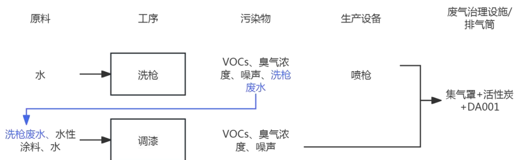
图 2-6 项目整改前洗枪、调漆工作流程图
