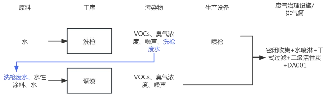
图 2-4 项目洗枪、调漆工作流程图
