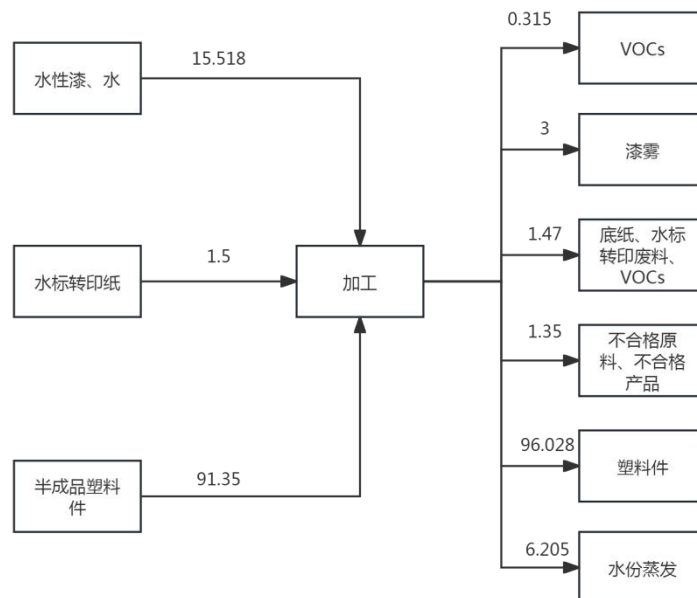
图2-2 物料平衡图 单位：t/a
