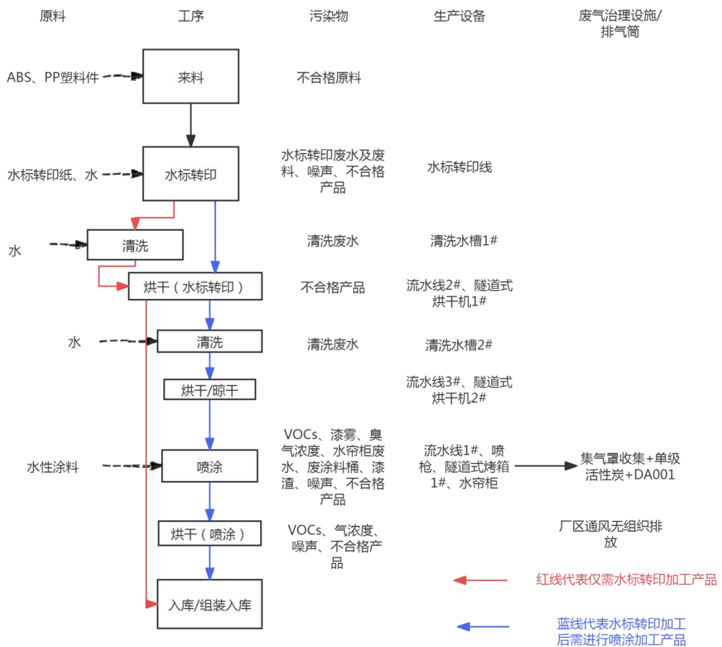
图 2-5 项目整改前主要工艺流程图
