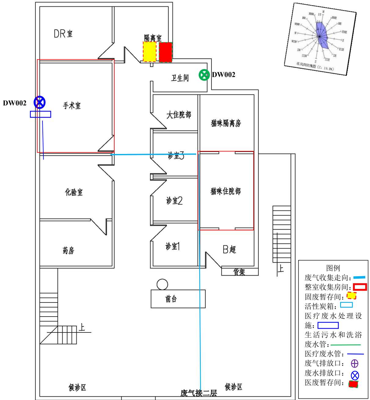
附图 3.1 项目平面布置图（首层）
