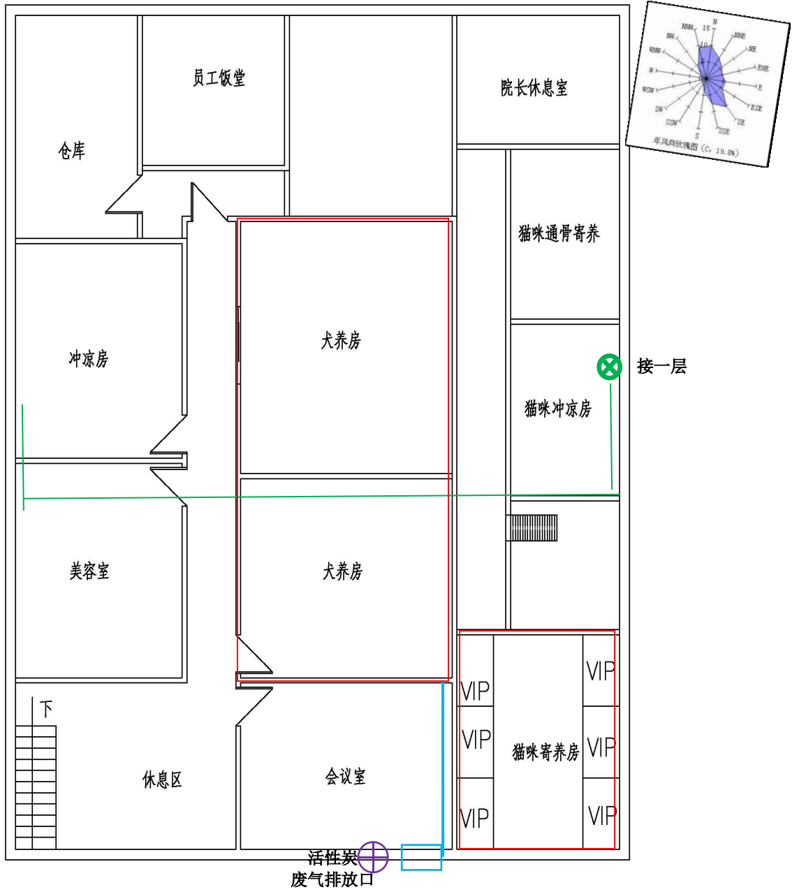
附图 3.2 项目平面布置图（二层）
