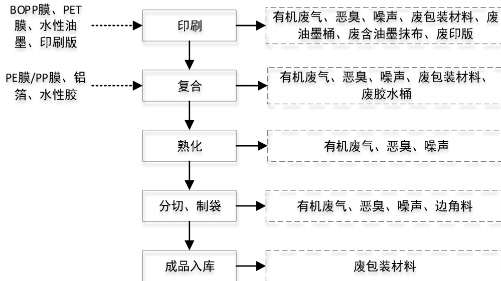
图 2-4 工艺流程及排污节点图
