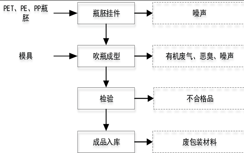
图 2-2 工艺流程及排污节点图
