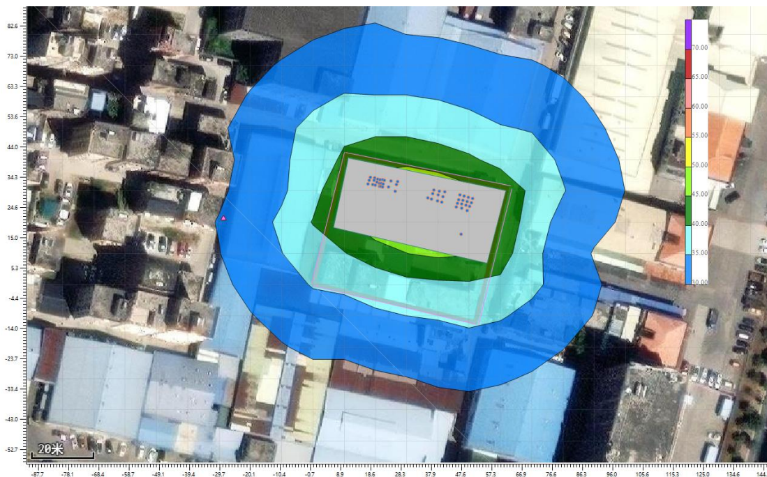
图 4-2 昼间噪声贡献值等值线示意图
