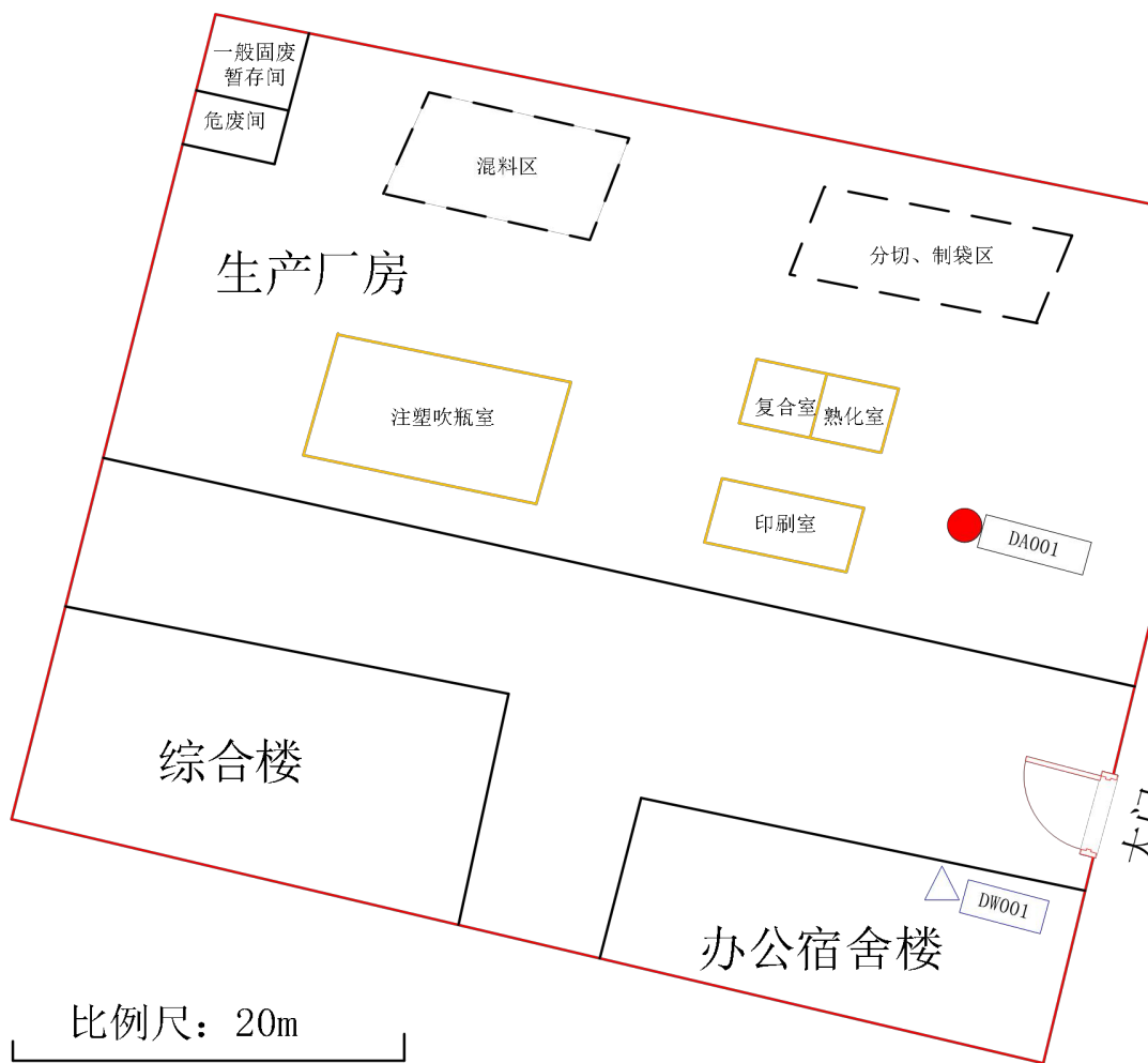
附图 4 项目厂区总平面布置图
