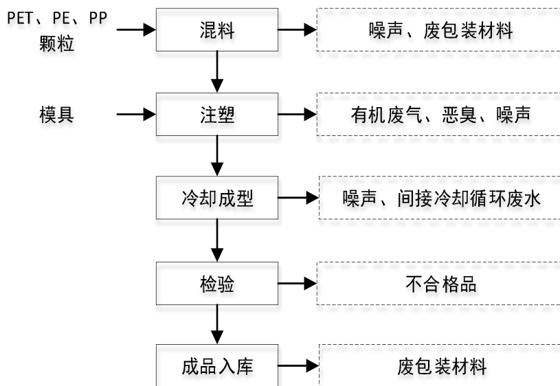
图 2-3 工艺流程及排污节点图
