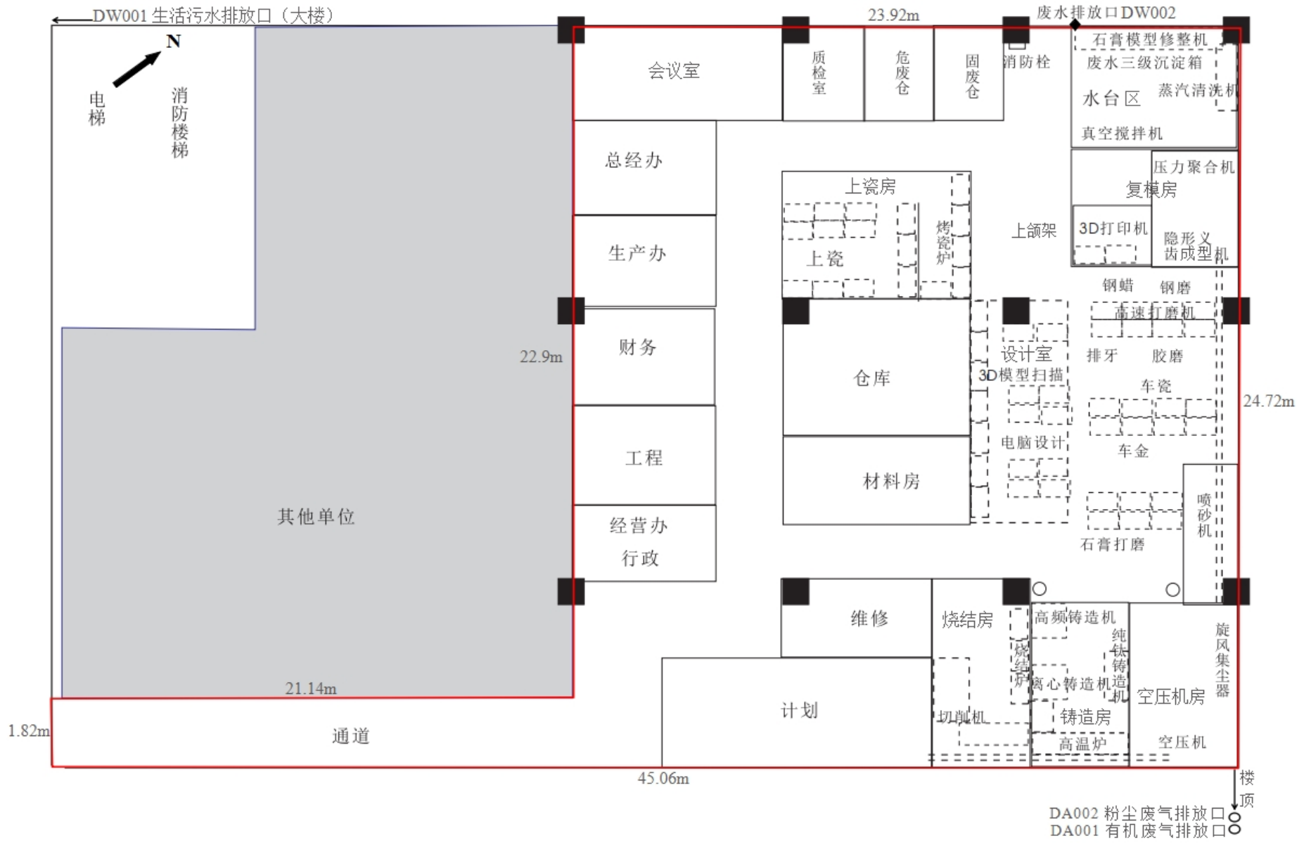
附图3 项目总平面布置图
