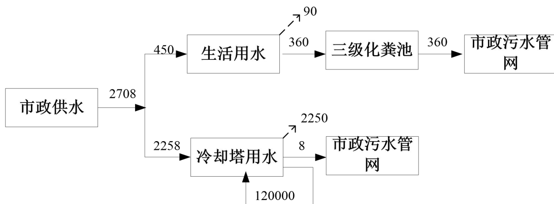
图 2-2 本项目水平衡图（单位：t/a）
