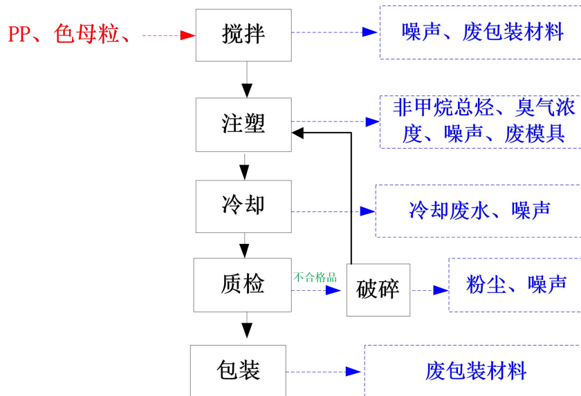
图 2-3 塑料盖工艺流程图
