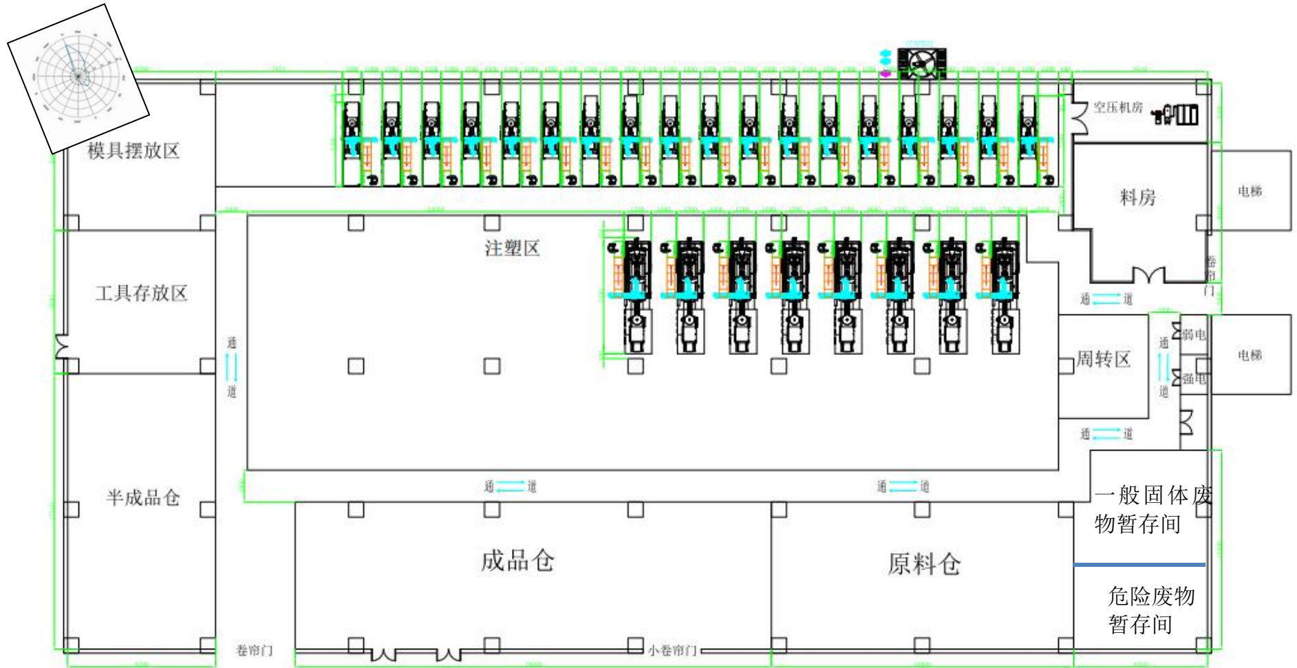
附图 5-2 项目 1F 平面图
