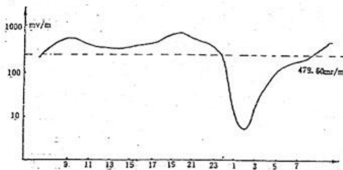
图2 综合场强——时间关系曲线图
