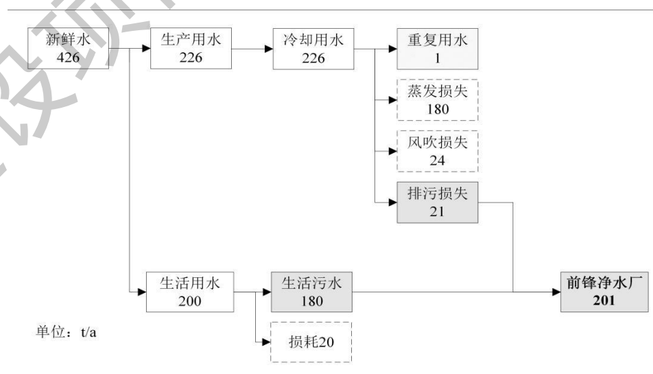
图 2-1 水平衡示意图
