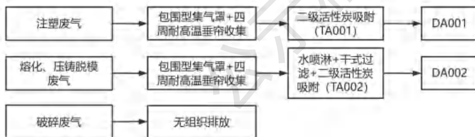
图 4-1 废气治理设施流程图
