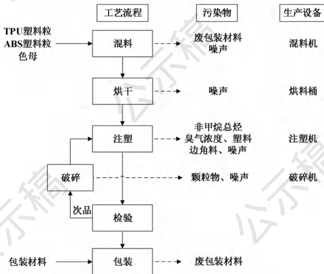
图 2-3 本项目音响密封圈生产工艺流程及产污环节图
