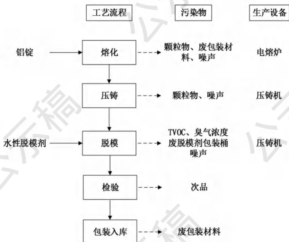
图 2-3 本项目音响骨架生产工艺流程及产污环节图
