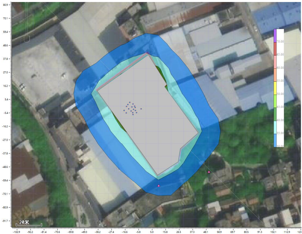
图 4-2 昼间噪声贡献值等值线示意图
