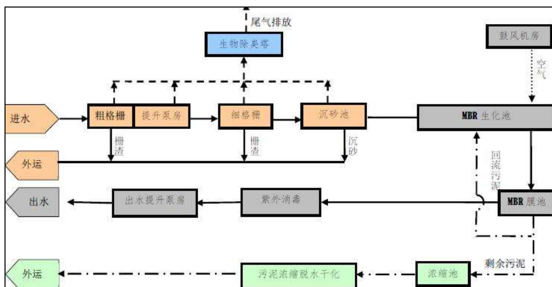
图4-5 新华污水处理厂工艺流程图
