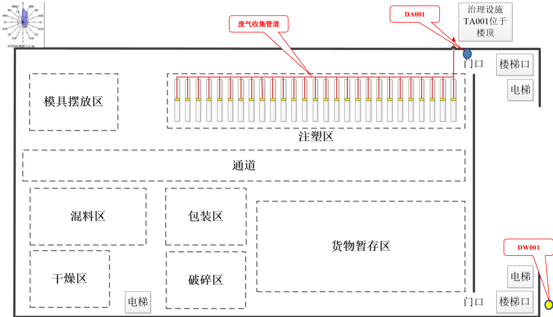
附图 4 建设项目 1F 平面布置图
