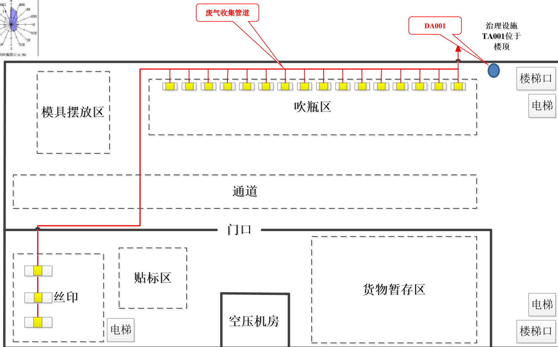
附图 6 建设项目 3F 平面布置图
