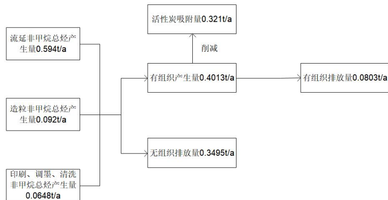
图 4-1 项目有机废气平衡图
