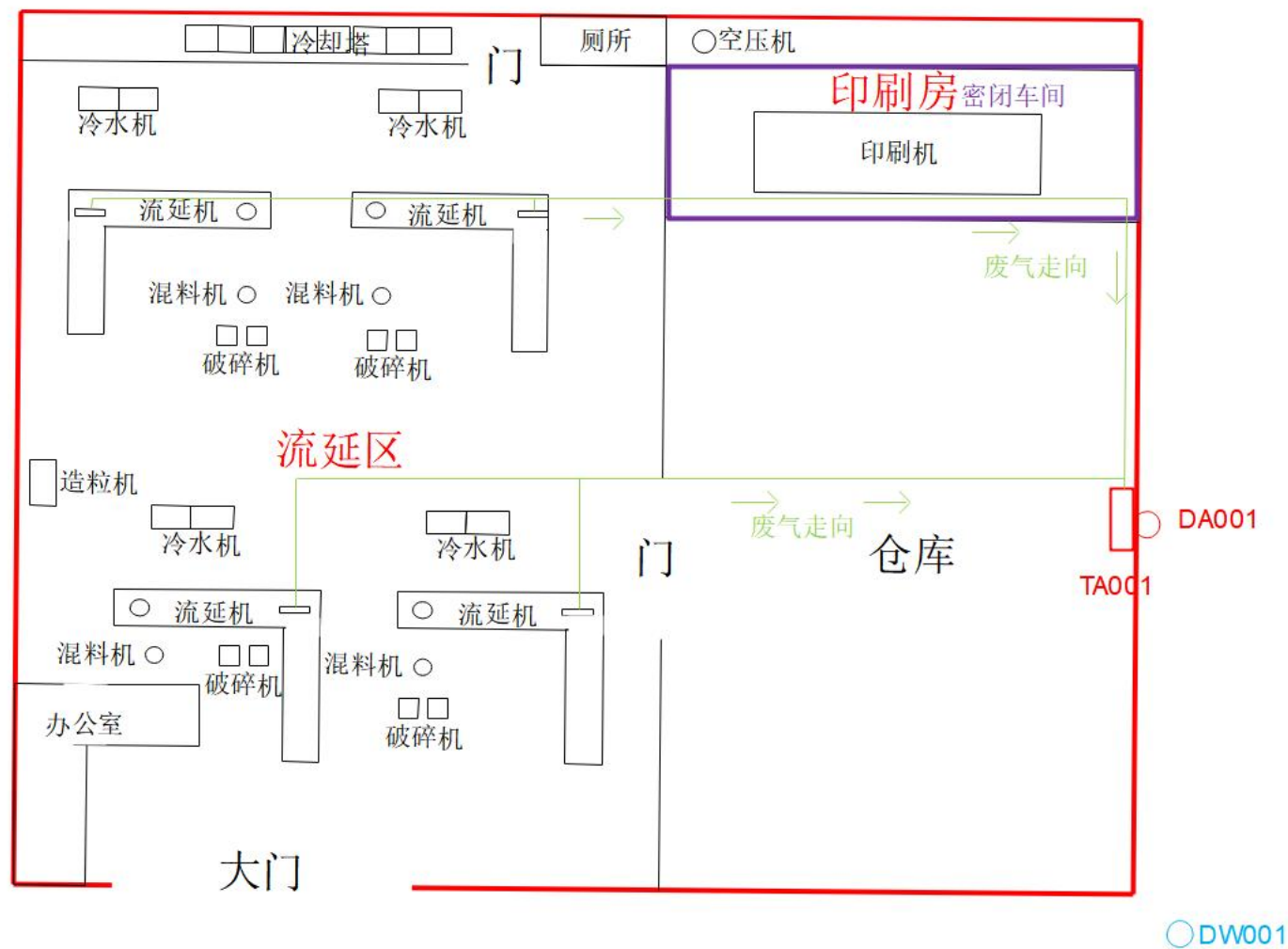
附图 4-2 项目生产厂房平面图
