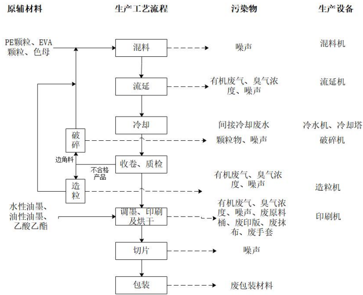
图 2-2 生产工艺流程
