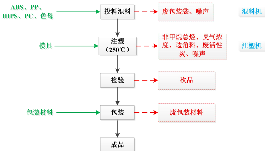
图 2-3 本项目音响塑料外壳生产工艺流程及产污环节图
