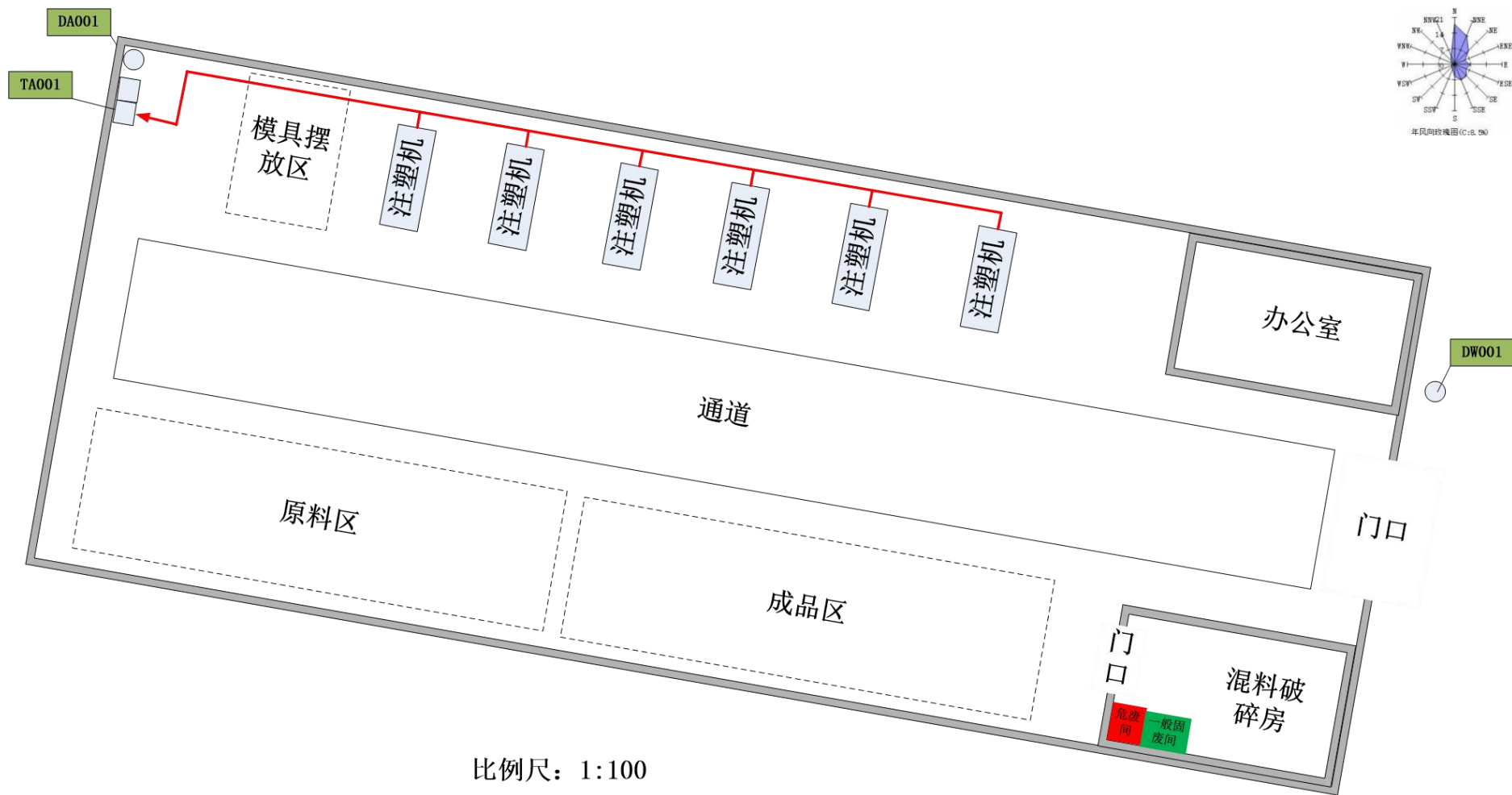
附图 4 建设项目总平面布置图
