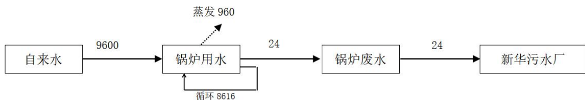
图 2-1 本项目水平衡图（单位：t/a）
