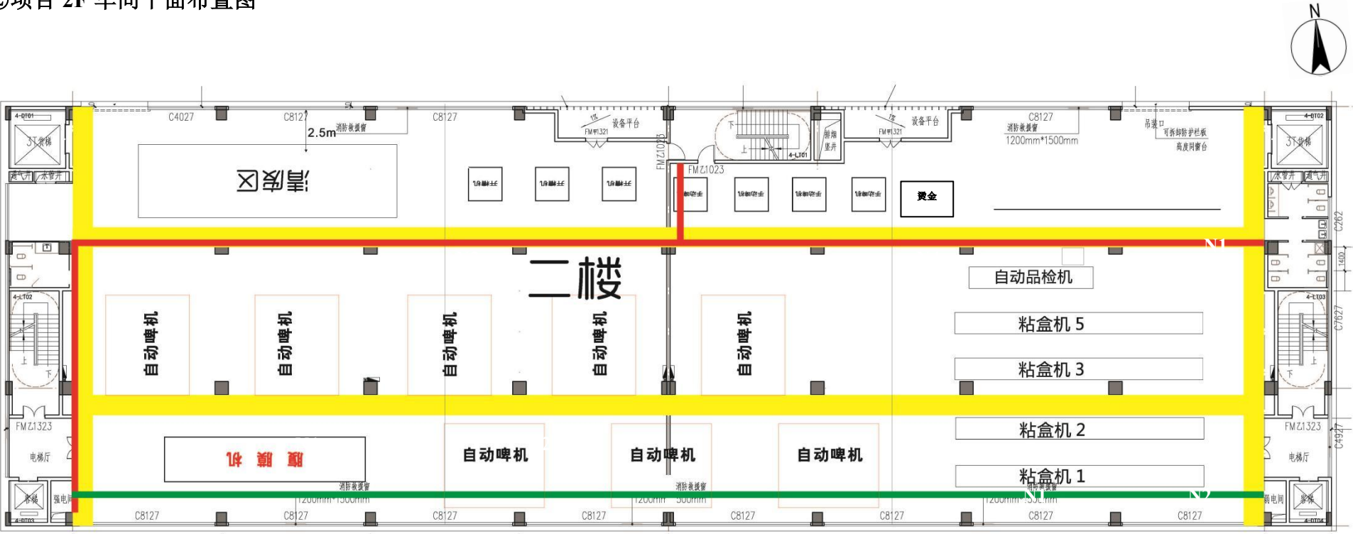
②项目 2F 车间平面布置图
