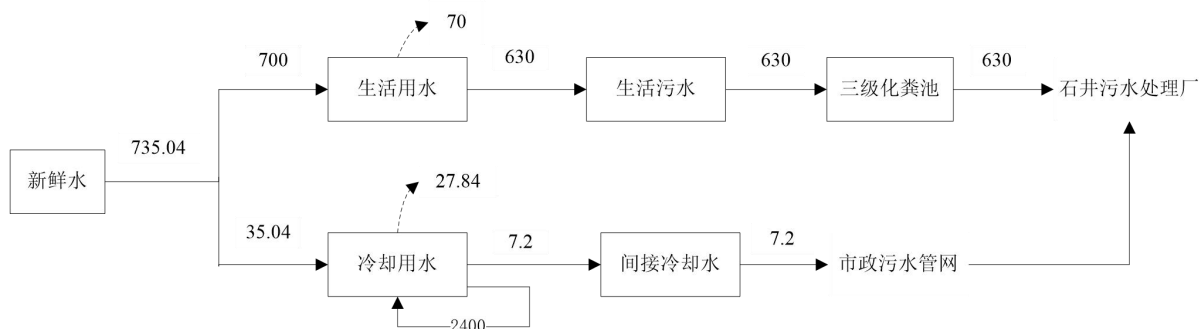
图1 本项目水平衡图 (m 3 /a)
