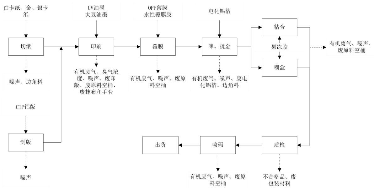
图2 本项目纸盒和礼品盒生产工艺流程及产污环节图
