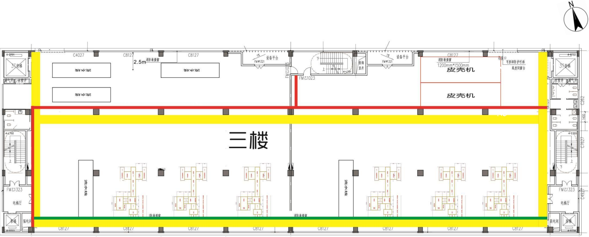
③项目 3F 车间平面布置图
