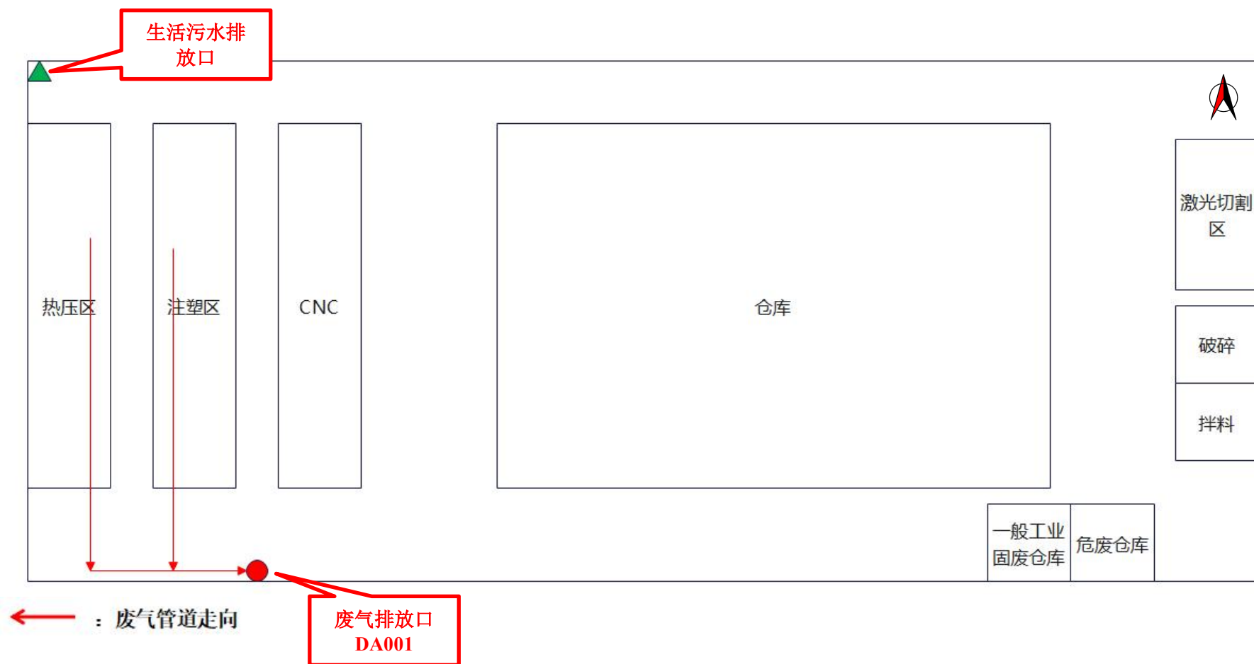
附图 5 项目厂区总平面布置图及废气收集管道走向图
