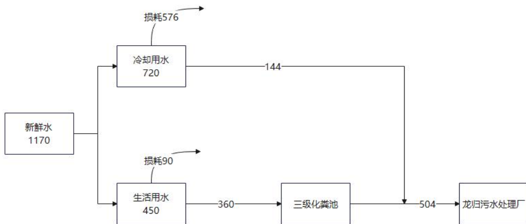
图 2 本项目水平衡图 (单位 m³/a)
