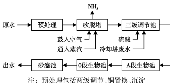
图 4 酞菁蓝生产废水处理工艺
