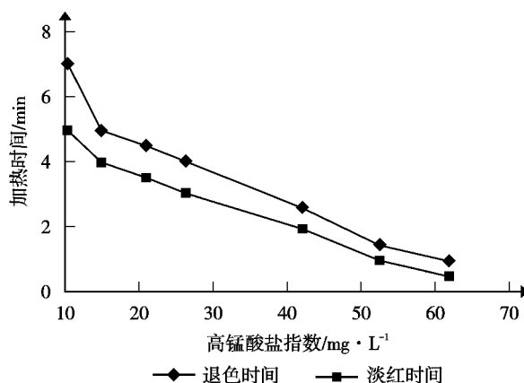
图 1 加热颜色变化时间与高锰酸盐指数的关系
