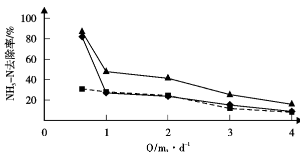
c. 流量变化对NH 3 -N去除率影响
