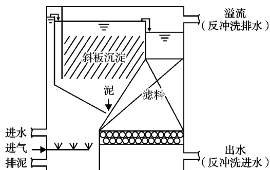
图 2 废水处理一体化装置示意
