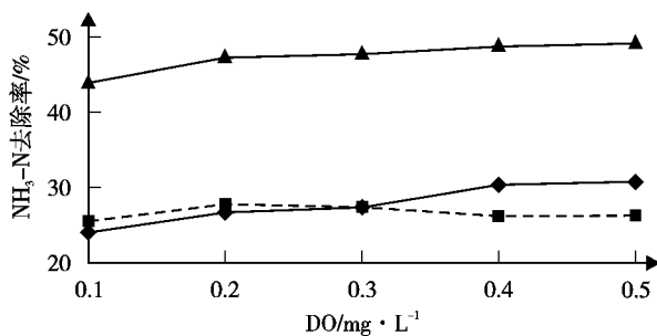
b. DO变化对NH 3 -N去除率影响
