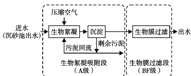
图 1 一体化装置废水处理工艺流程
