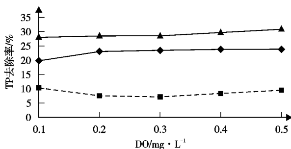
c. DO变化对TP去除率影响
