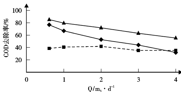
b. 流量变化对COD去除率影响
