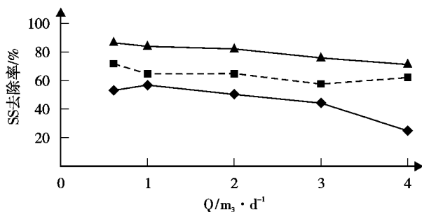
a. 流量变化对SS去除率影响
