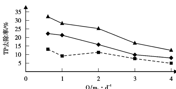
d. 流量变化对TP去除率影响
