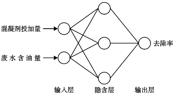
图 1 BP 神经网络模型
