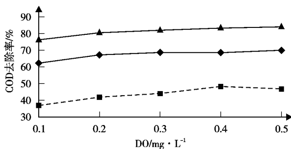
a. DO变化对COD去除率影响
