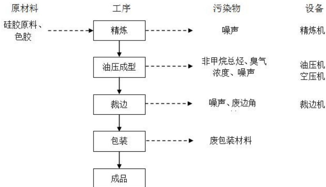
图 2-2 本项目运营期整体工作流程图
