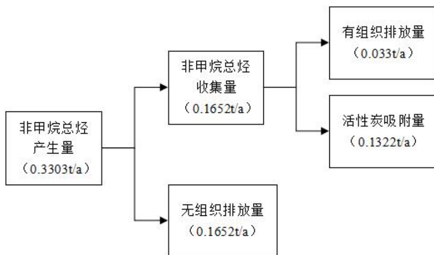
图 4-1 项目非甲烷总烃平衡图
