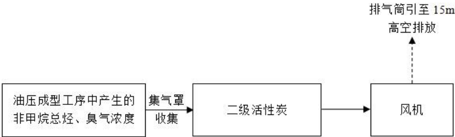
图 4-2 二级活性炭吸附装置处理工艺流程图
