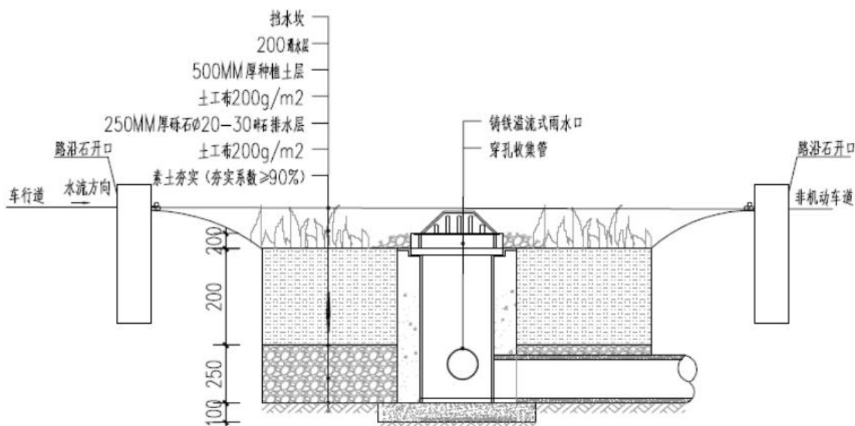
图 6 下沉式绿地构造示意图
