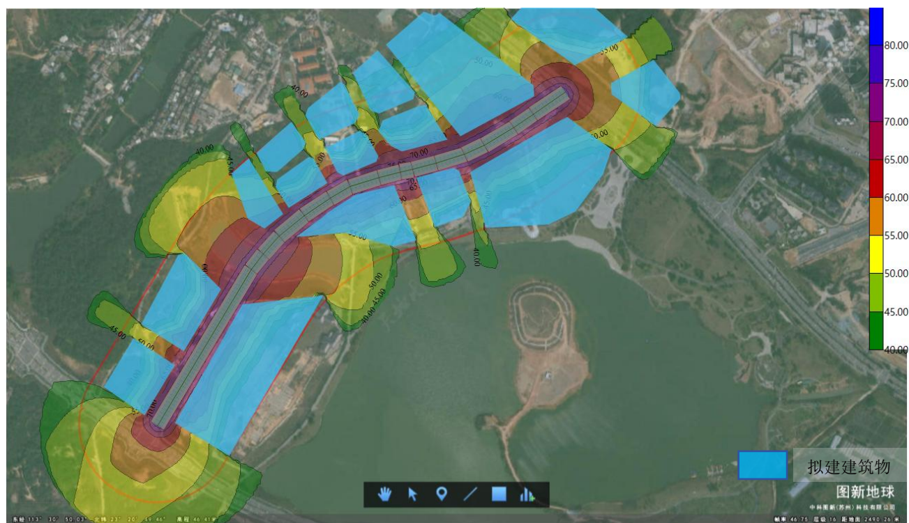
图 5.2-8 2032 年昼间等声级线图
