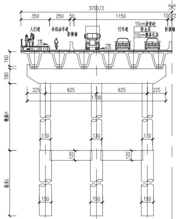
图 2 桥梁立面图
