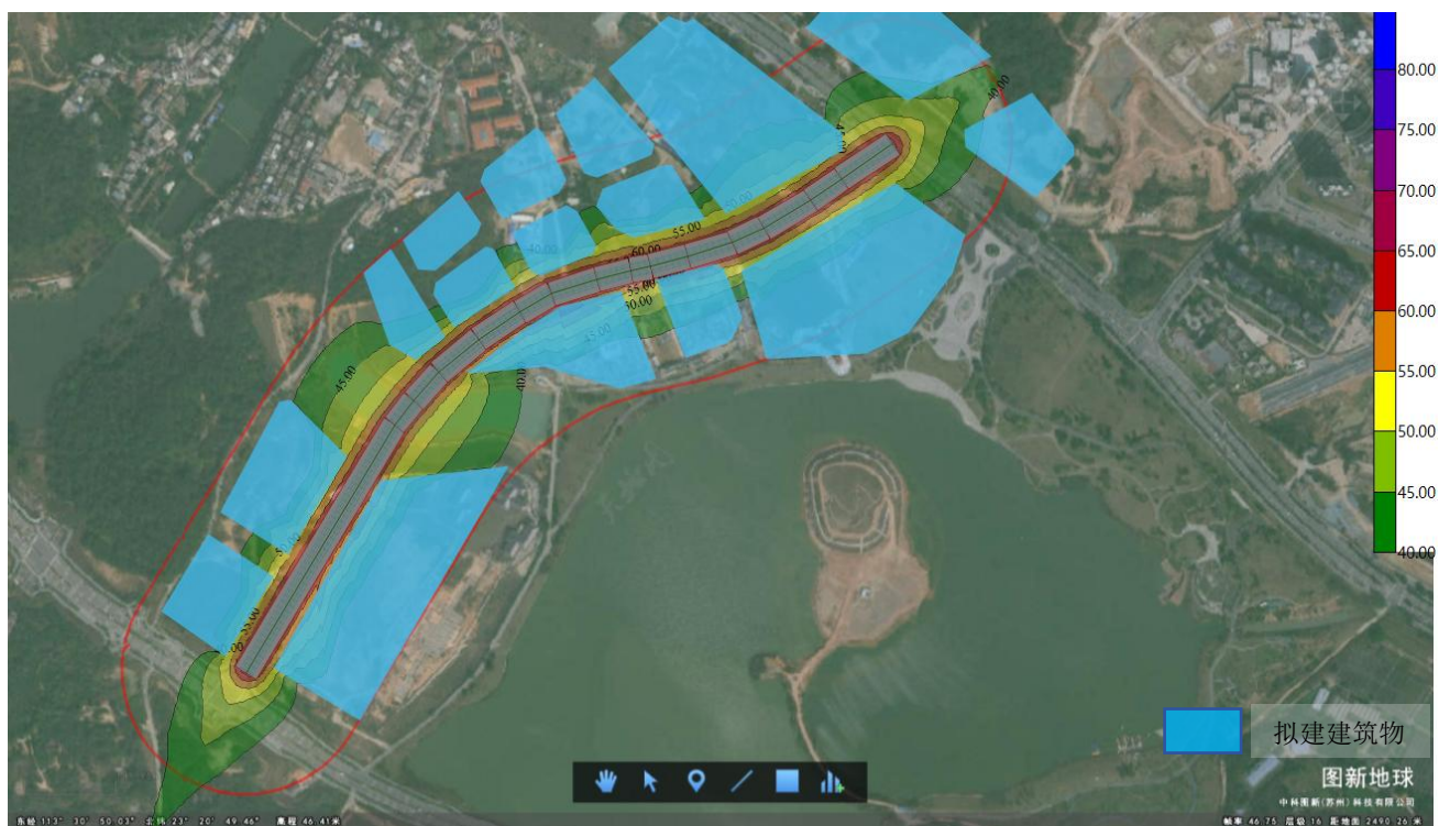
图 5.2-9 2032 年夜间等声级线图
