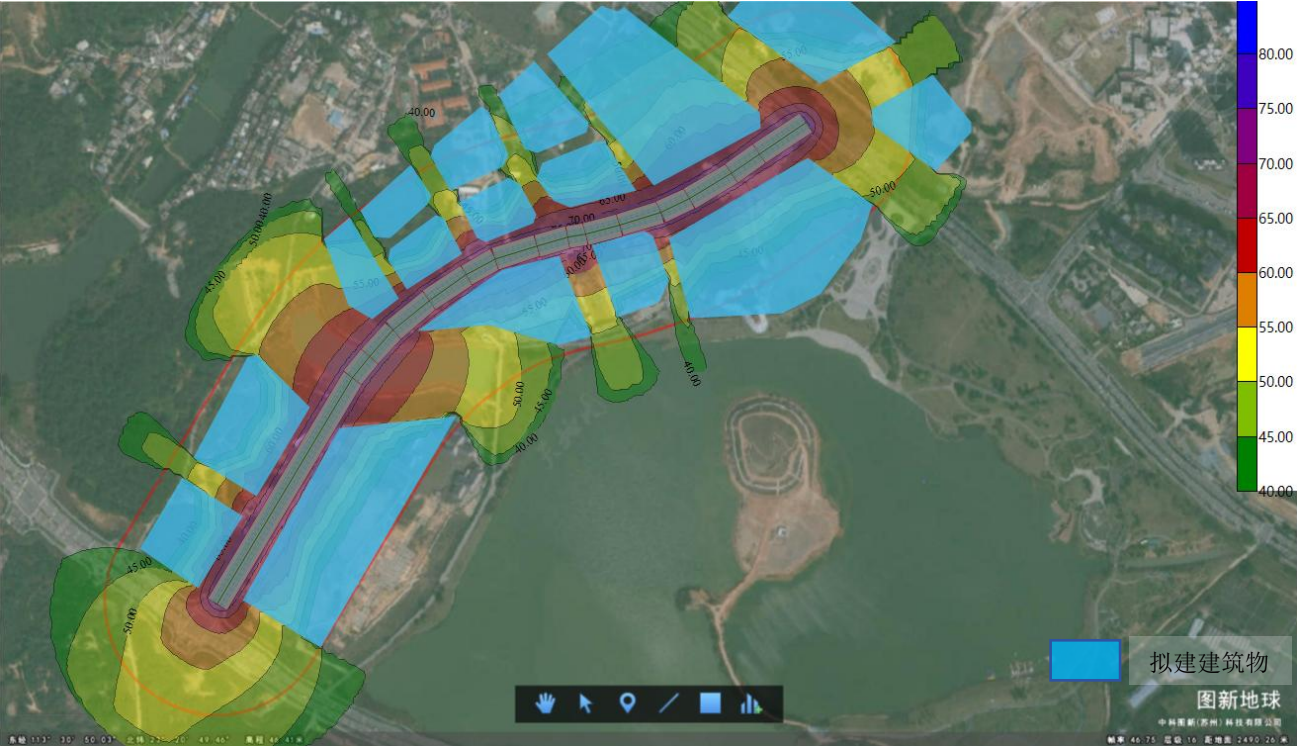
图 5.2- 6 2026 年昼间等声级线图
