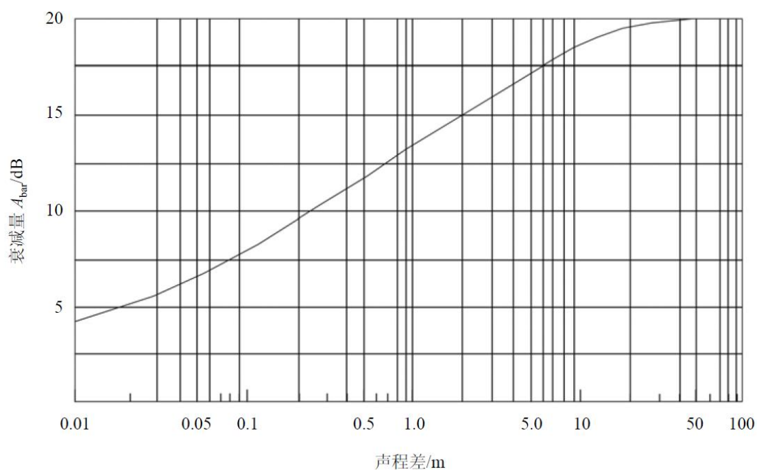
图 5.2-3 噪声衰减量 L_{\bar{a}} 与声程差 \delta 关系曲线 ( f=500\text{Hz} )
