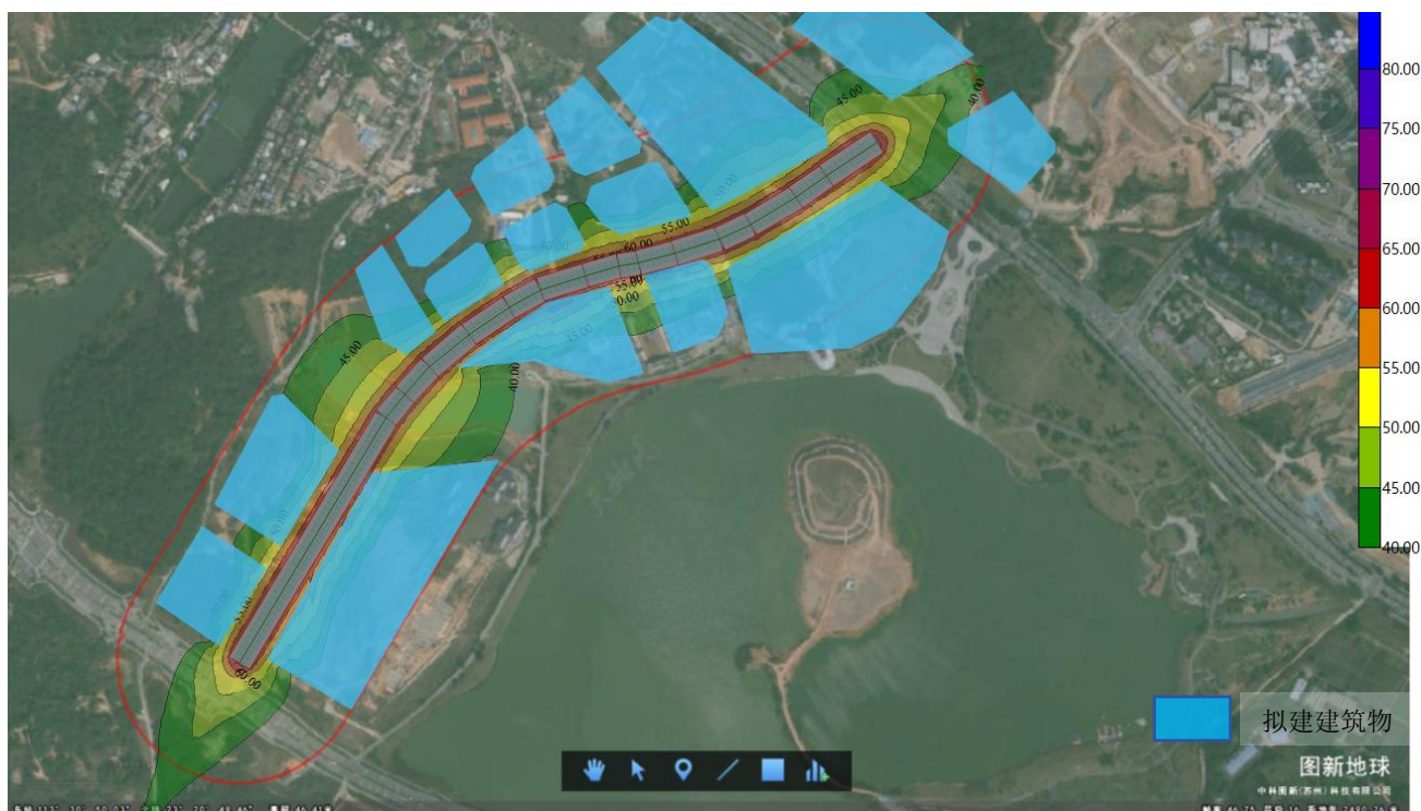
图 5.2-11 2040 年夜间等声级线图
