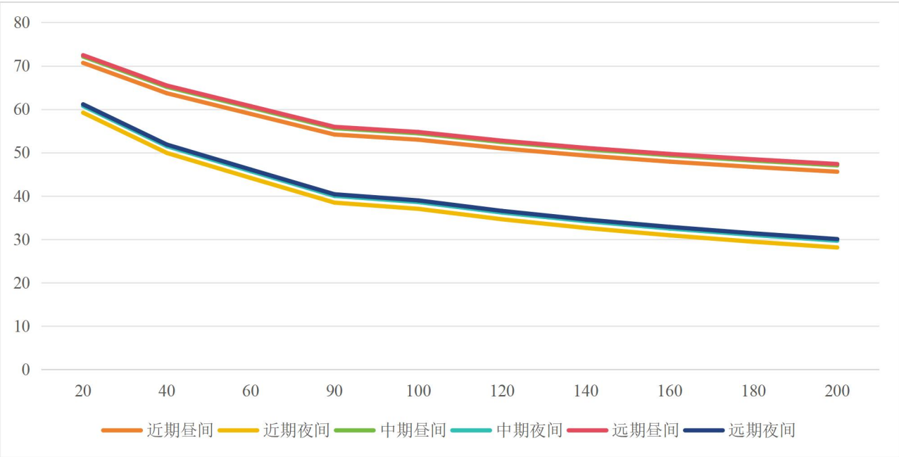
图 5.2- 5 本项目横断面噪声衰减预测示意图
