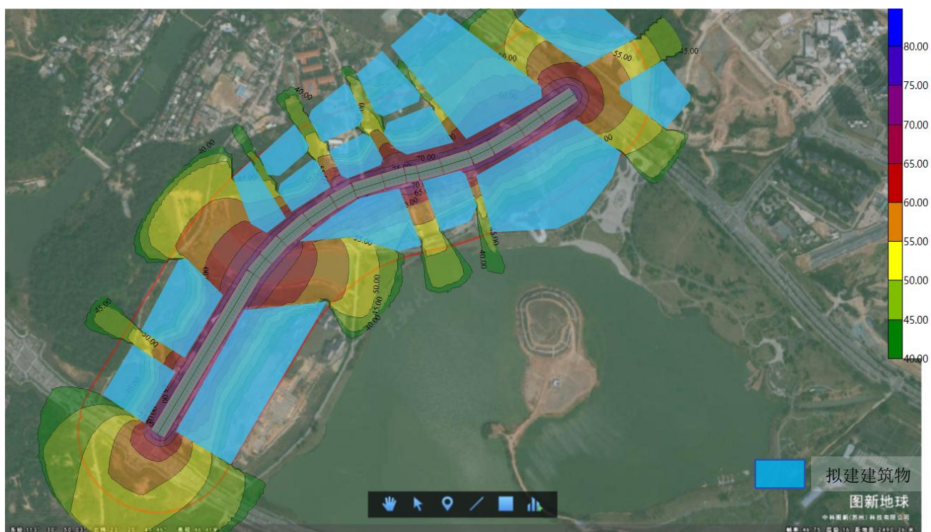
图 5.2-10 2040 年昼间等声级线图
