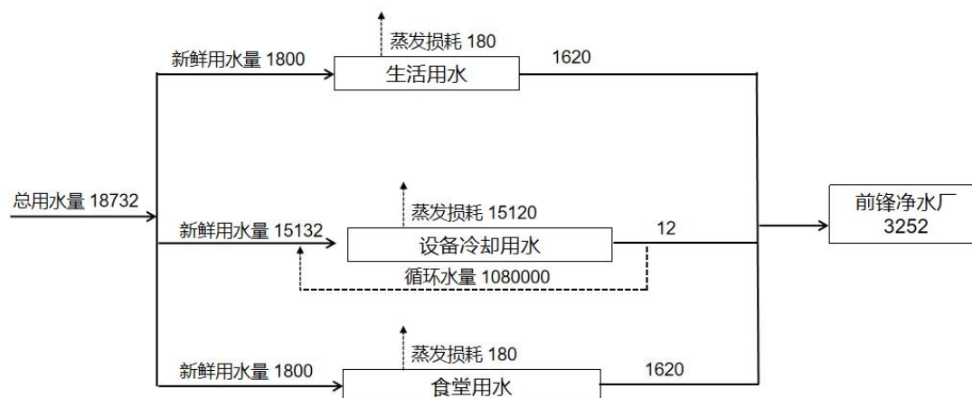
图 2-2 项目用水量平衡图, t/a
