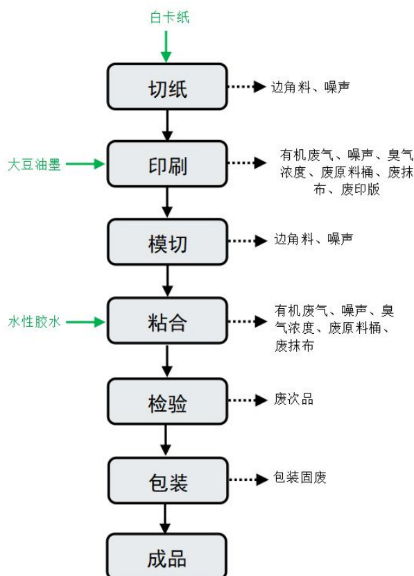
图 2-2 化妆品彩盒生产工艺流程及产污环节图
