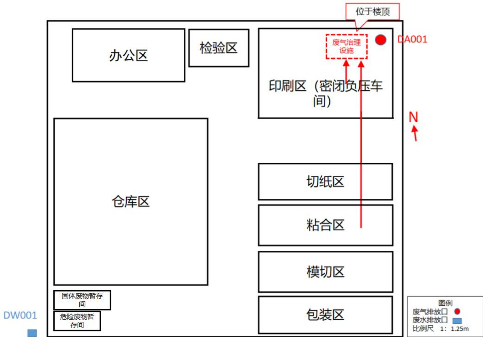
附图3 项目车间布置平面图
