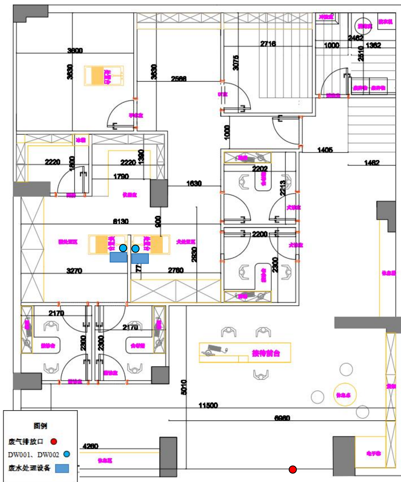
一楼平面图
