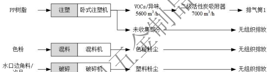
图 4-2 废气收集、治理和排放汇总示意图
