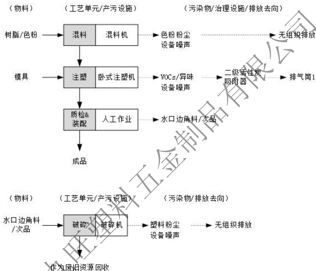
图 2-2 工艺流程和产污环节示意图
