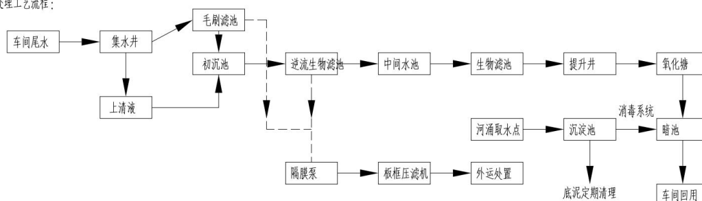
图 4-1 养殖废水处理工艺流程图
