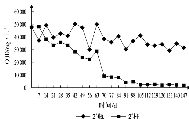
图 5 2# 瓶和 2# 柱渗滤液的降解曲线
