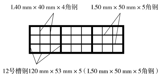
图3 站房地面(屋面、正立面)钢框架示意
