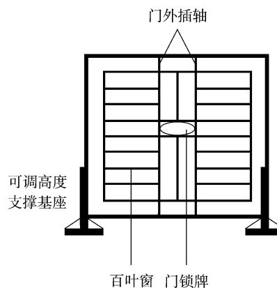
图 2 M2 及站房侧立面示意
