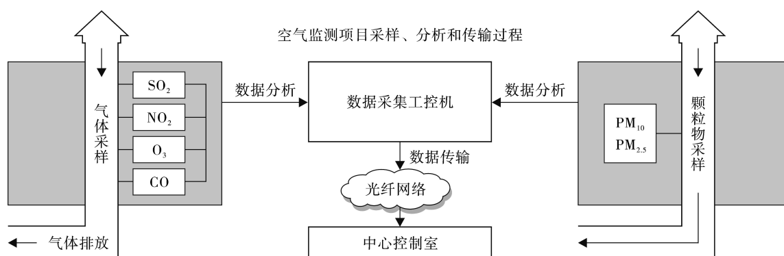
图 11 子站系统工作示意
