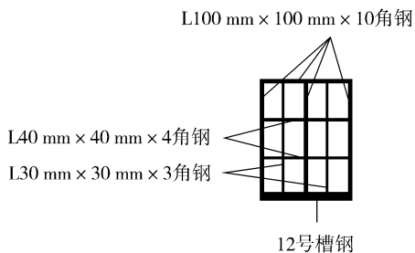
图4 站房侧立面钢框架示意
