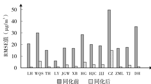
图6 同站站点 SO 2 同化前后 RMSE 值对比
