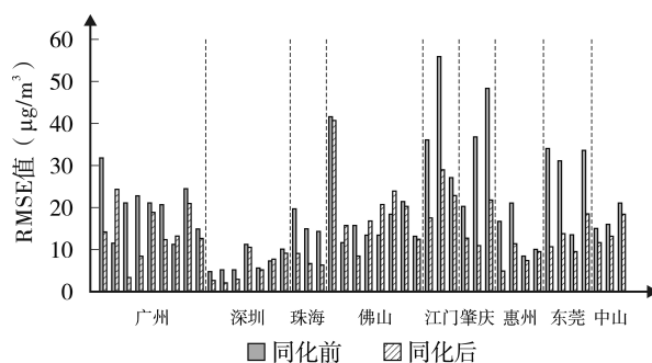
图7 检验站点 SO 2 同化前后 RMSE 值对比
