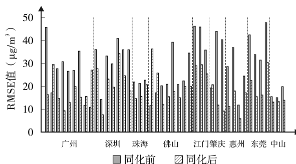
图3 检验站点 \text{NO}_2 同化前后RMSE值对比
