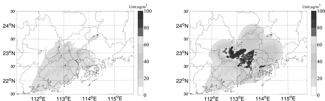
图 12 PM_{10} 同化前后月均浓度分布(左:同化前;右:同化后)
