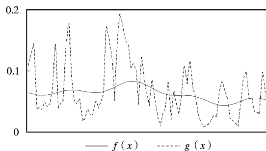
图2 2007年1月1日~3月31日二氧化硫的实测值 g(x) 和模型计算值 f(x)
