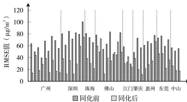
图11 检验站点 PM 10 同化前后 RMSE 值对比
