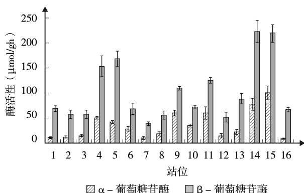
图2 红树林不同站位沉积物样品 \alpha -葡萄糖苷酶和 \beta -葡萄糖苷酶的活性比较
