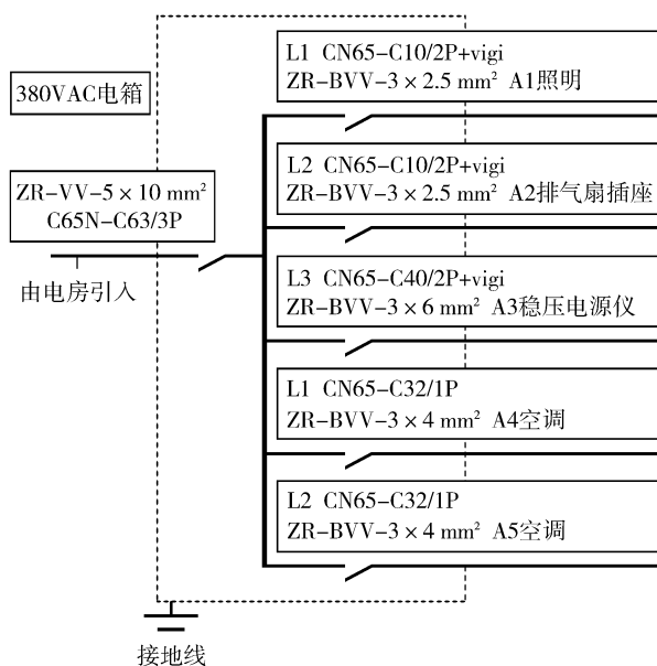
图5 配电系统示意
