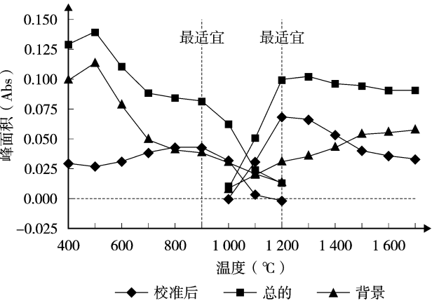
图2 加入 5 g/L 的磷酸二氢铵所得的灰化原子化图
