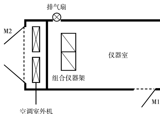
图 1 站房平面示意
