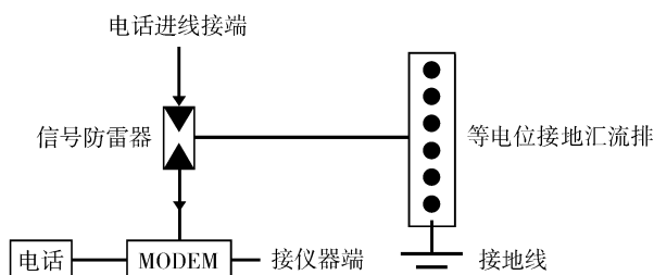
图7 信号系统保护示意
