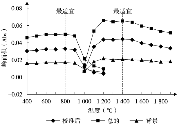
图3 加入 10 g/L(左图)和加入 2 g/L(右图)的硝酸铵所得的灰化原子化
