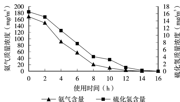
图 3 新型微生物除臭剂对垃圾渗滤主要恶臭气体去除效果
