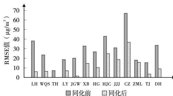
图2 同化站点 \text{NO}_2 同化前后RMSE值对比
