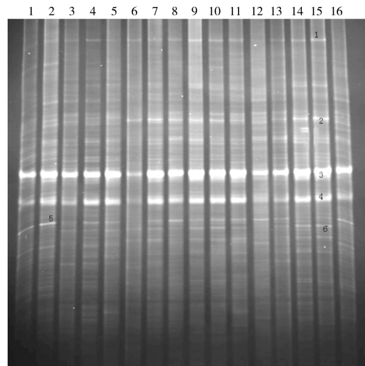
图 1 红树林沉积物不同站位细菌的 DGGE 指纹图谱
