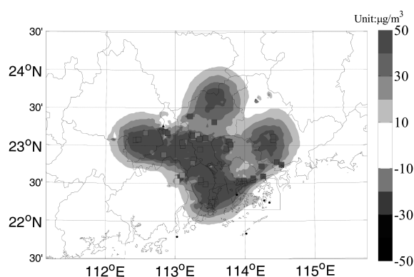
图 13 检验站点 PM_{10} 同化分析增量与模式误差对比
