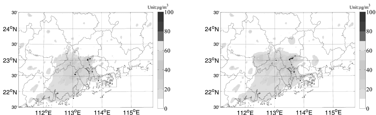
图8 SO 2 同化前后月均浓度分布(左:同化前;右:同化后)
