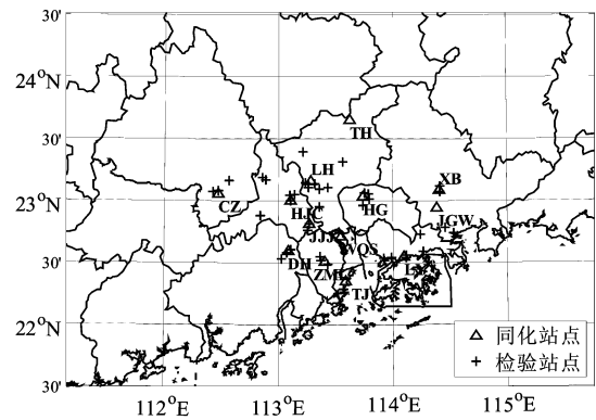
图 1 粤港珠三角区域空气监控网络站点(同化站点)及珠三角省控站点(检验站点)位置示意
