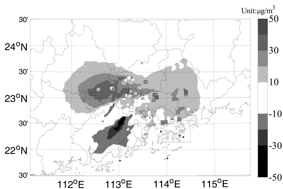
图5 检验站点 NO 2 同化分析增量与模式误差对比
