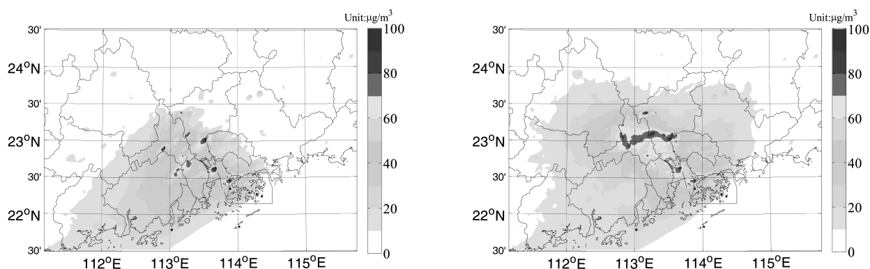
图4 NO 2 同化前后月均浓度分布(左:同化前;右:同化后)
