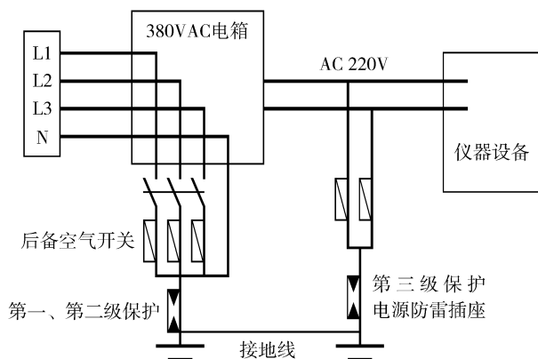
图6 交流电源系统保护示意
