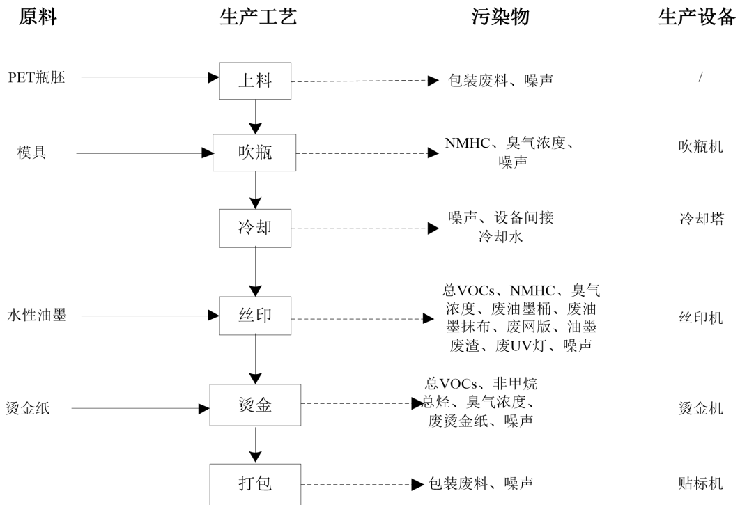
图 4 项目工艺流程及产污节点图
