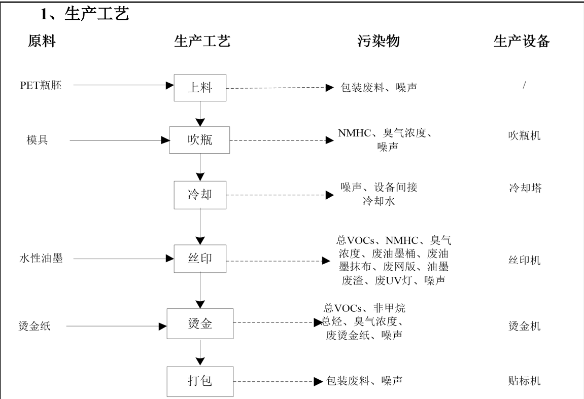
图3 塑料瓶身生产工艺流程及产污环节图
