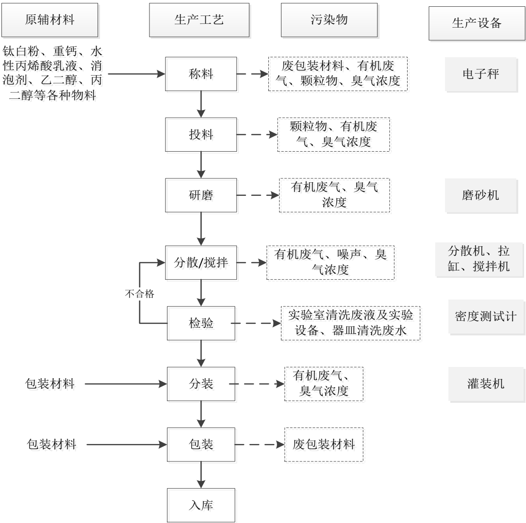
图 2-3 生产工艺流程图
