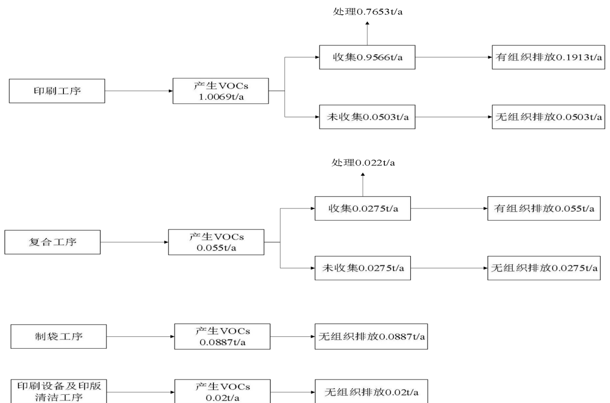
图 2-1 项目 VOCs 平衡图
