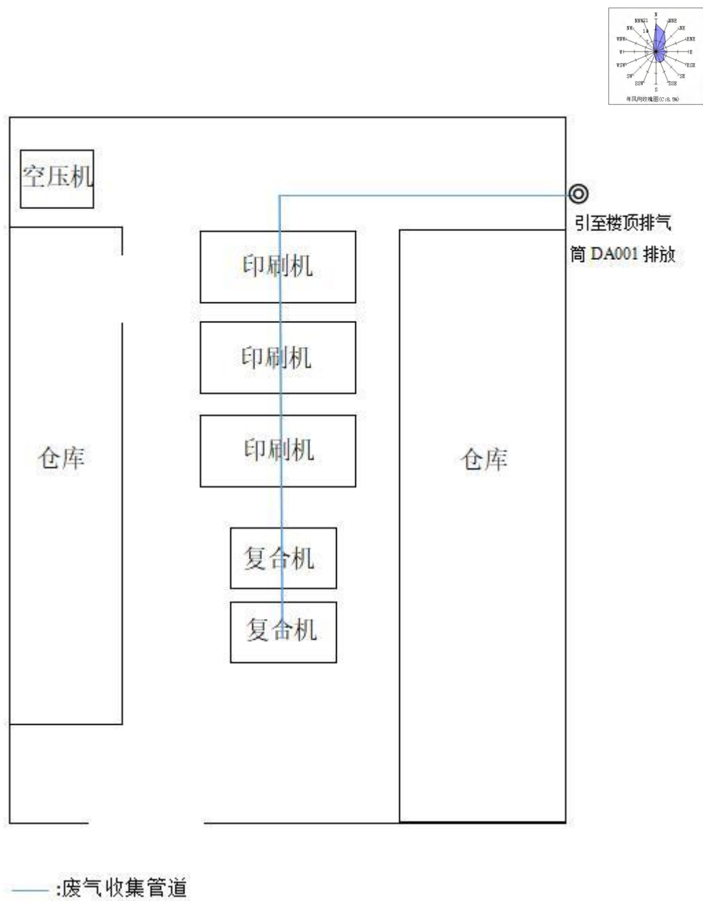
附图 6 项目第 1 层平面布置图
