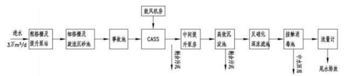
图 4-5 四涌西污水处理厂治理工艺流程图
