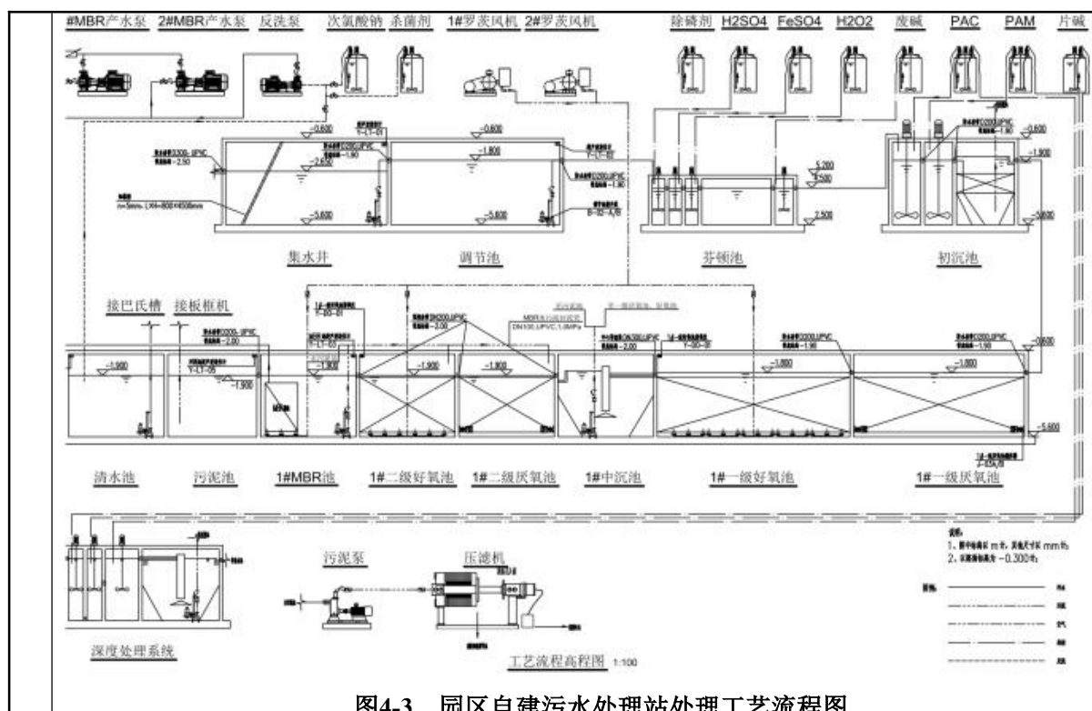
图4-3 园区自建污水处理站处理工艺流程图
