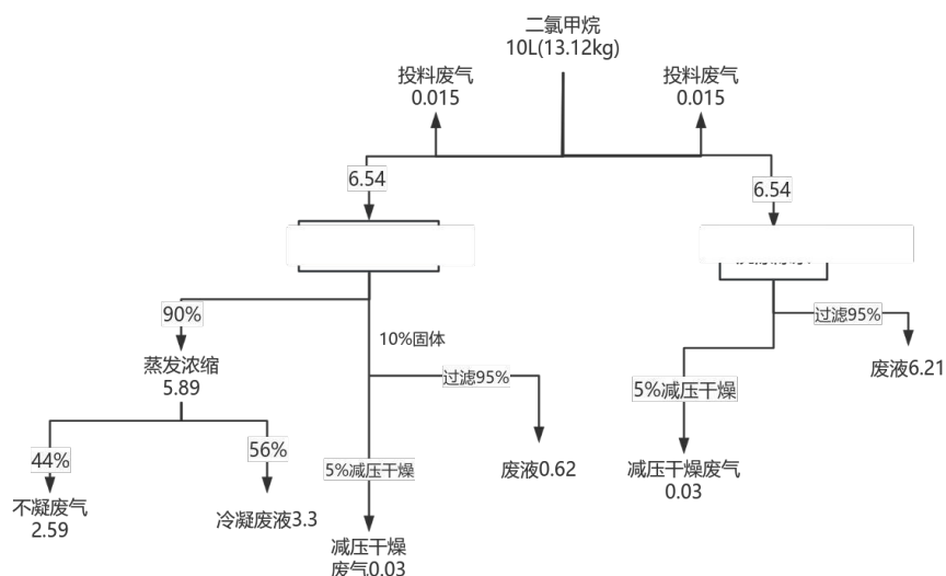
图 2-2 工艺部二氯甲烷物料平衡图 (kg/a)
