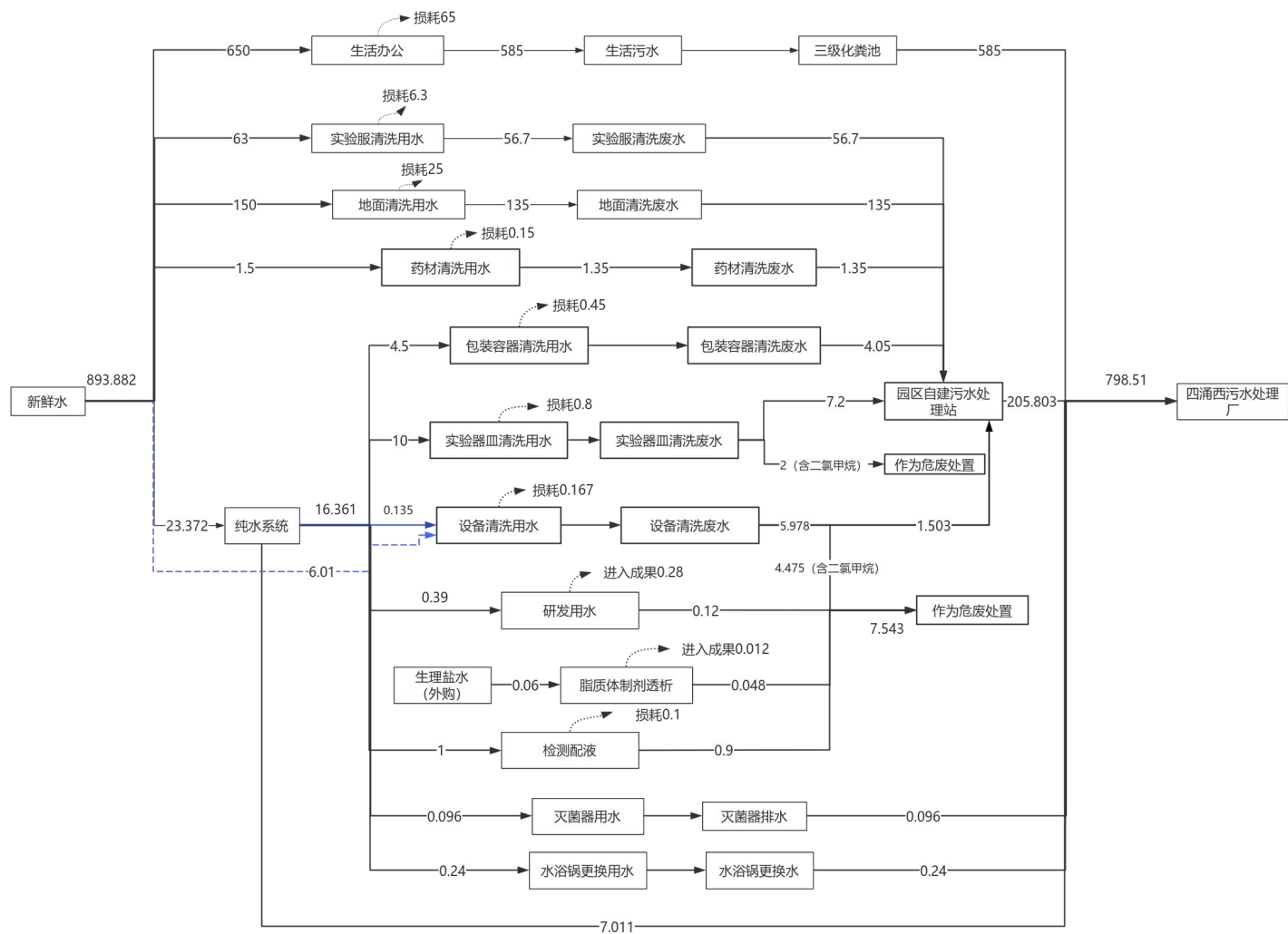
图 2-1 水平衡图（远期）（t/a）
