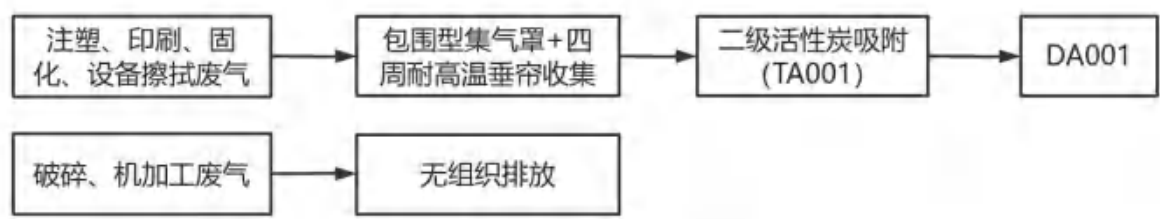
图 4-1 废气治理设施流程图
