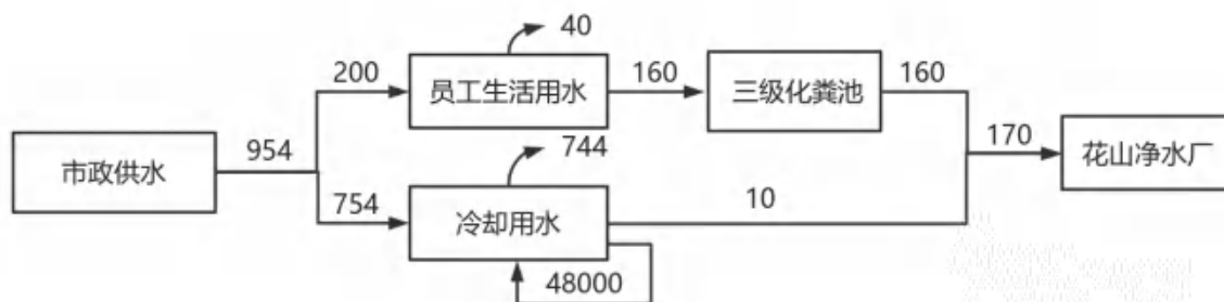
图 2-1 本项目水平衡图 (单位 m³/a)
