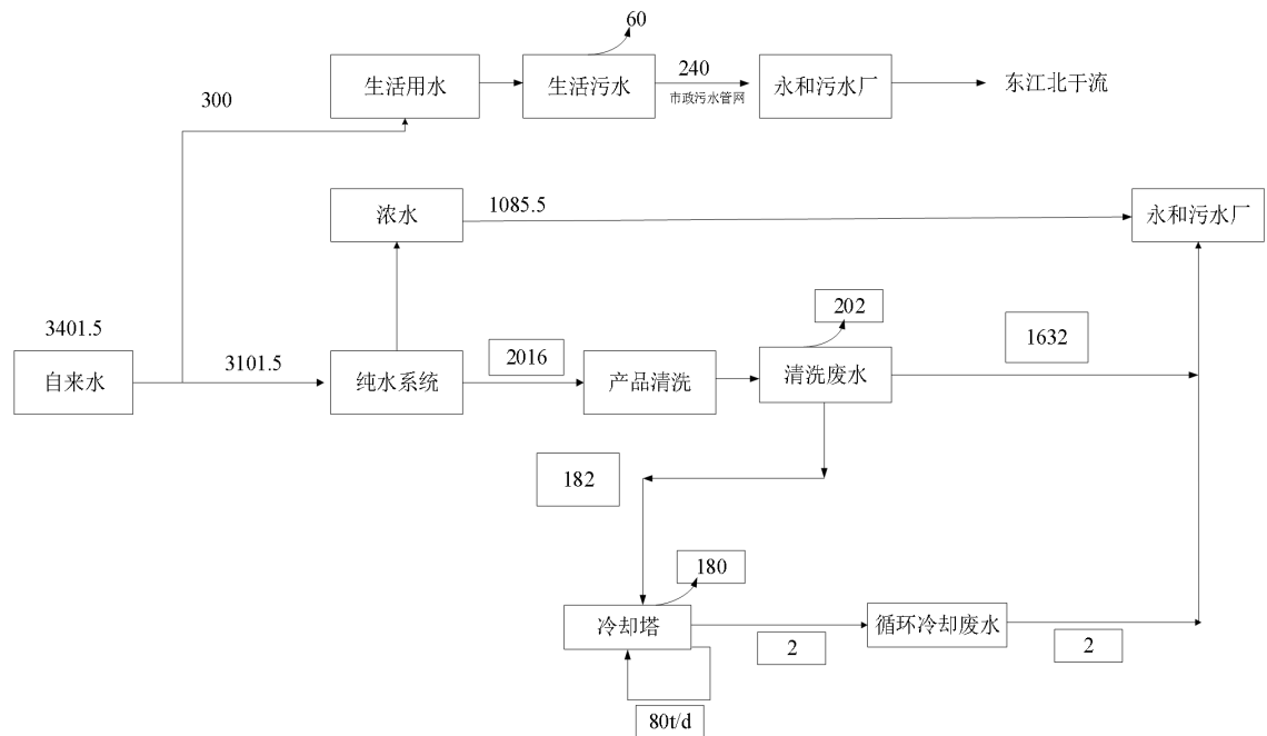
图 2-2 项目迁扩建后水平衡图 ( \text{t/a} )
