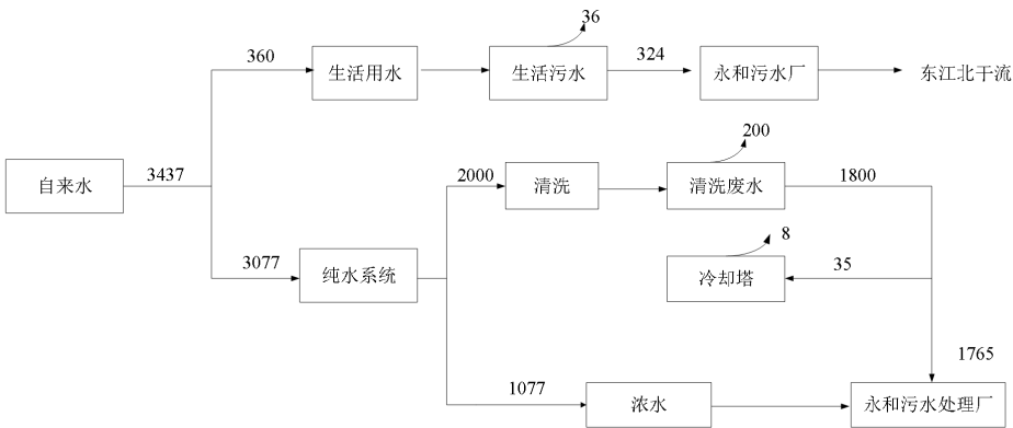
图 2-1 迁扩建前项目水平衡图（m 3 /a）
