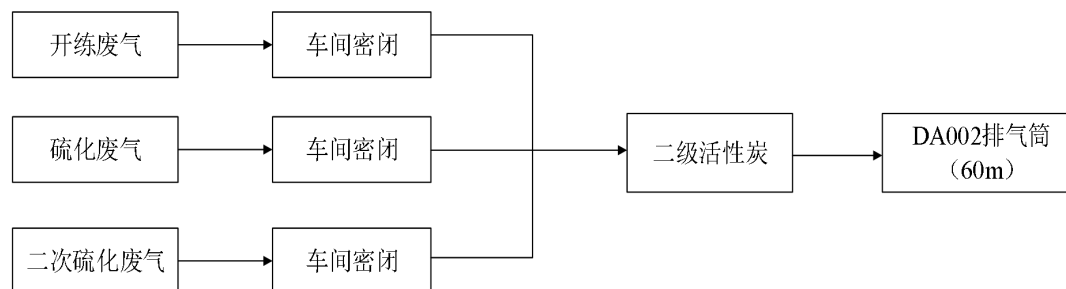
图 4-2 开炼、硫化成型、二次硫化废气处理工艺流程图
