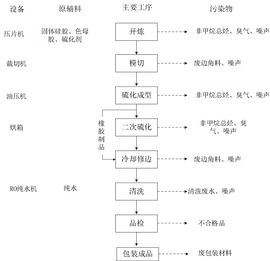
图 2-4 橡胶/硅胶制品生产工艺流程图
