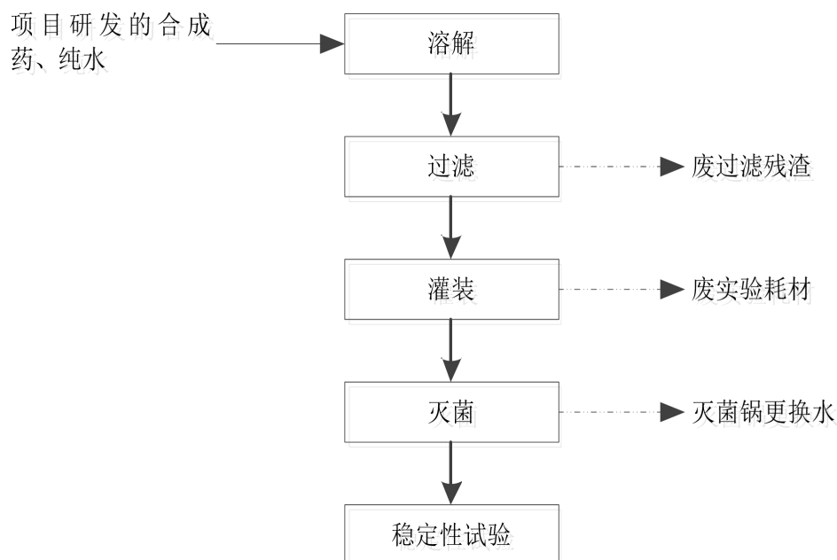
图 2-6 项目制剂工艺流程及产污环节图
