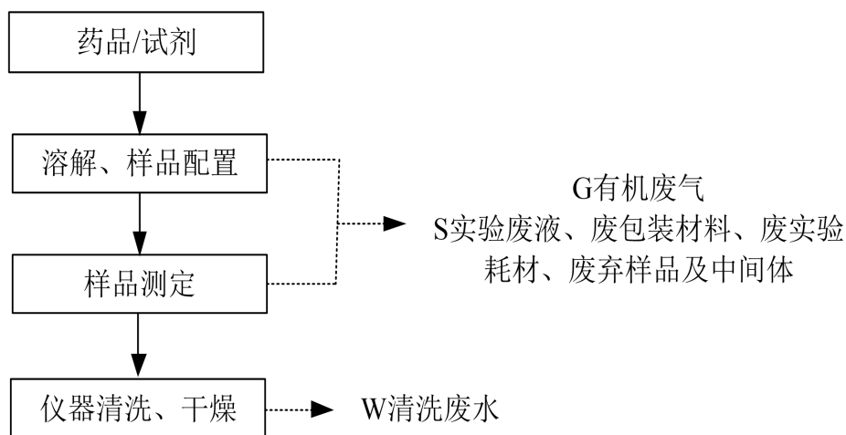
图 2-4 分析检测流程及产物节点图
