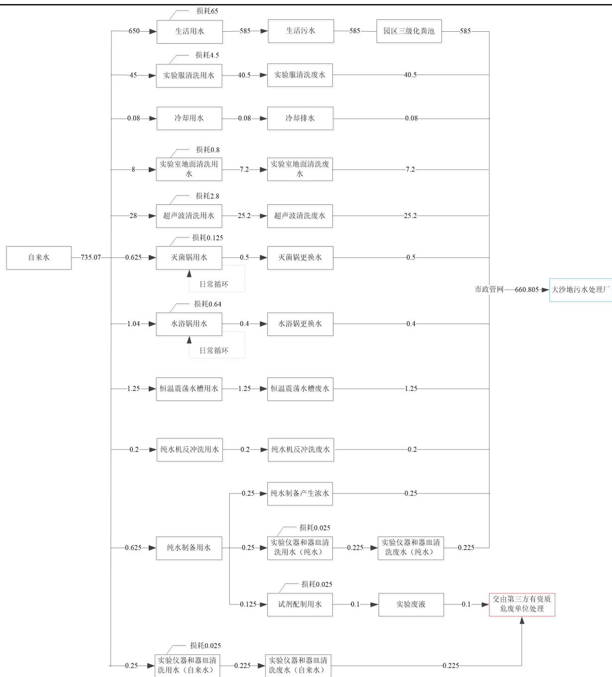
图2-2 项目水平衡图（单位：t/a）
