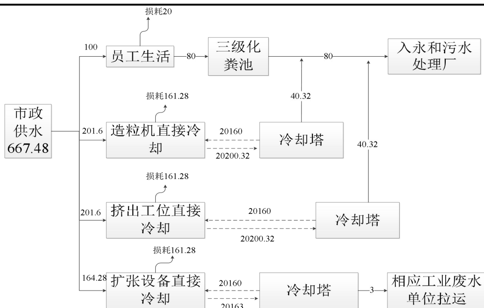
图 2-2 本项目水平衡图 (单位 m³/a)
