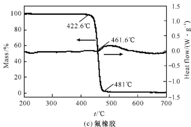
图1 镁粉、硝酸钠和氟橡胶的TG-DTA 曲线
