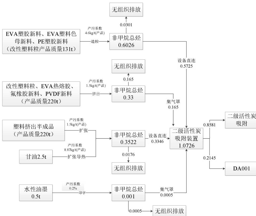
图 2-3 本项目有机废气平衡图 (单位 t/a)
