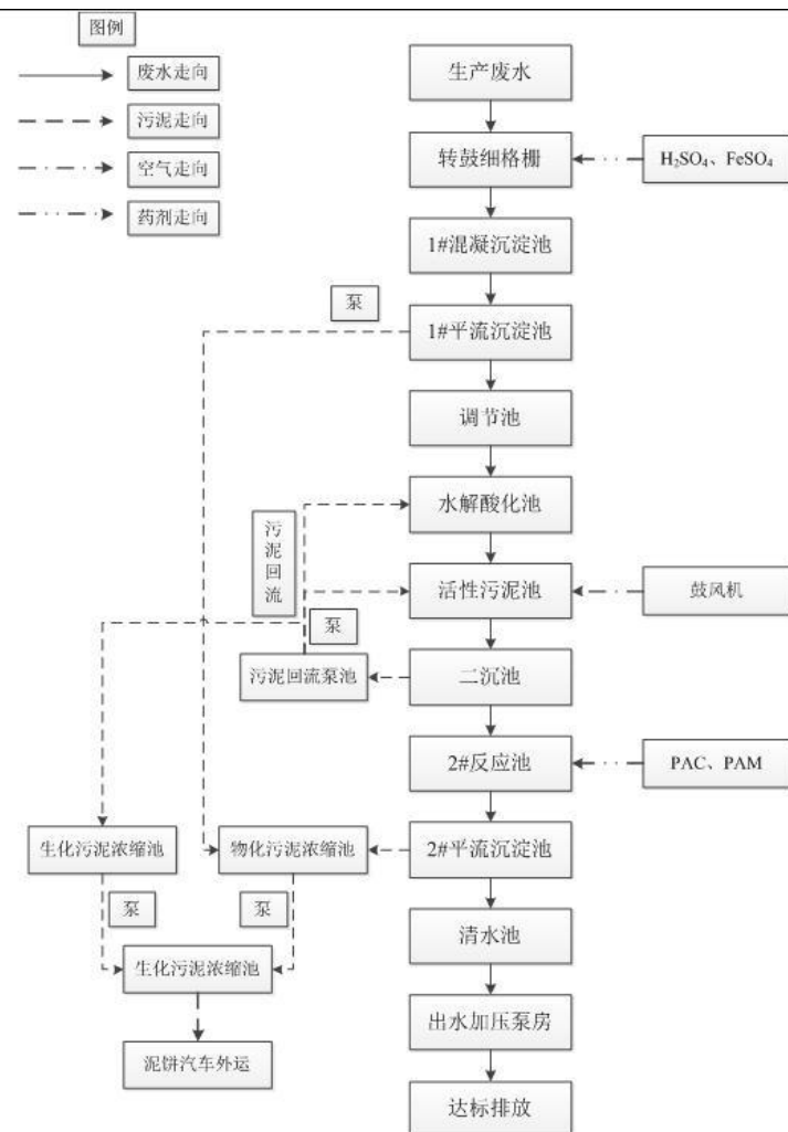
图 4-4 永和污水处理厂三期污水处理工艺流程图
