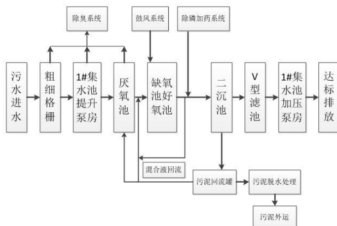
图 4-3 永和污水处理厂一、二期污水处理工艺流程图
