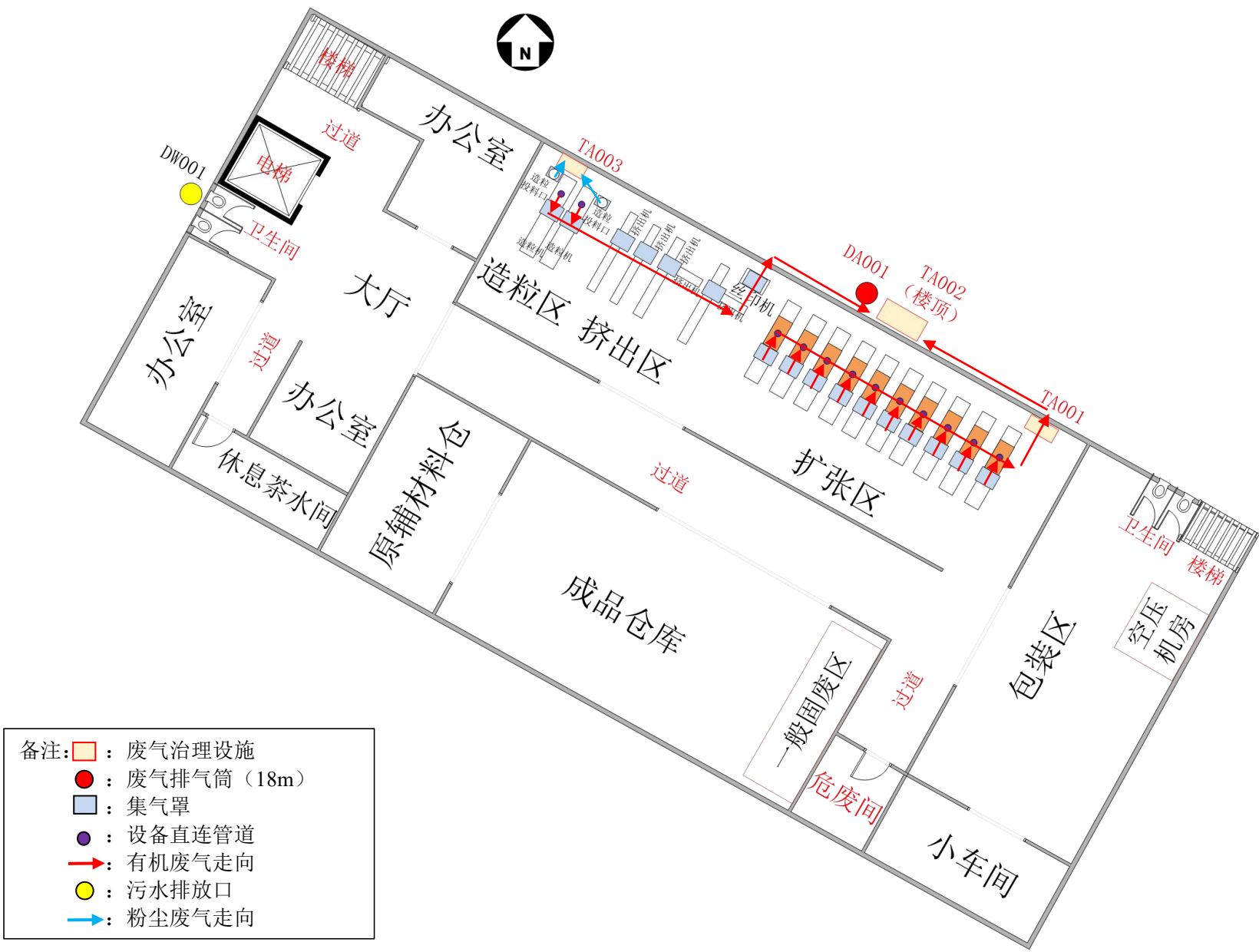
附图 4 建设项目平面布置图
