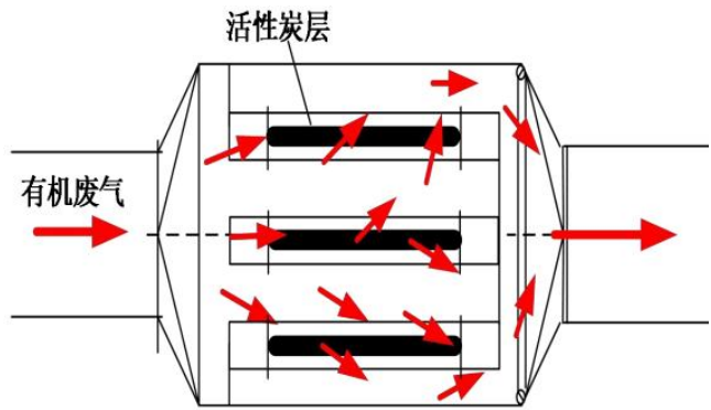
图 4-5 本项目活性炭箱设计图
