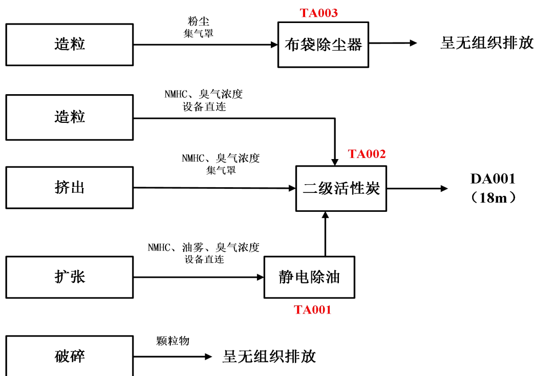
图 4-1 项目废气走向示意图
