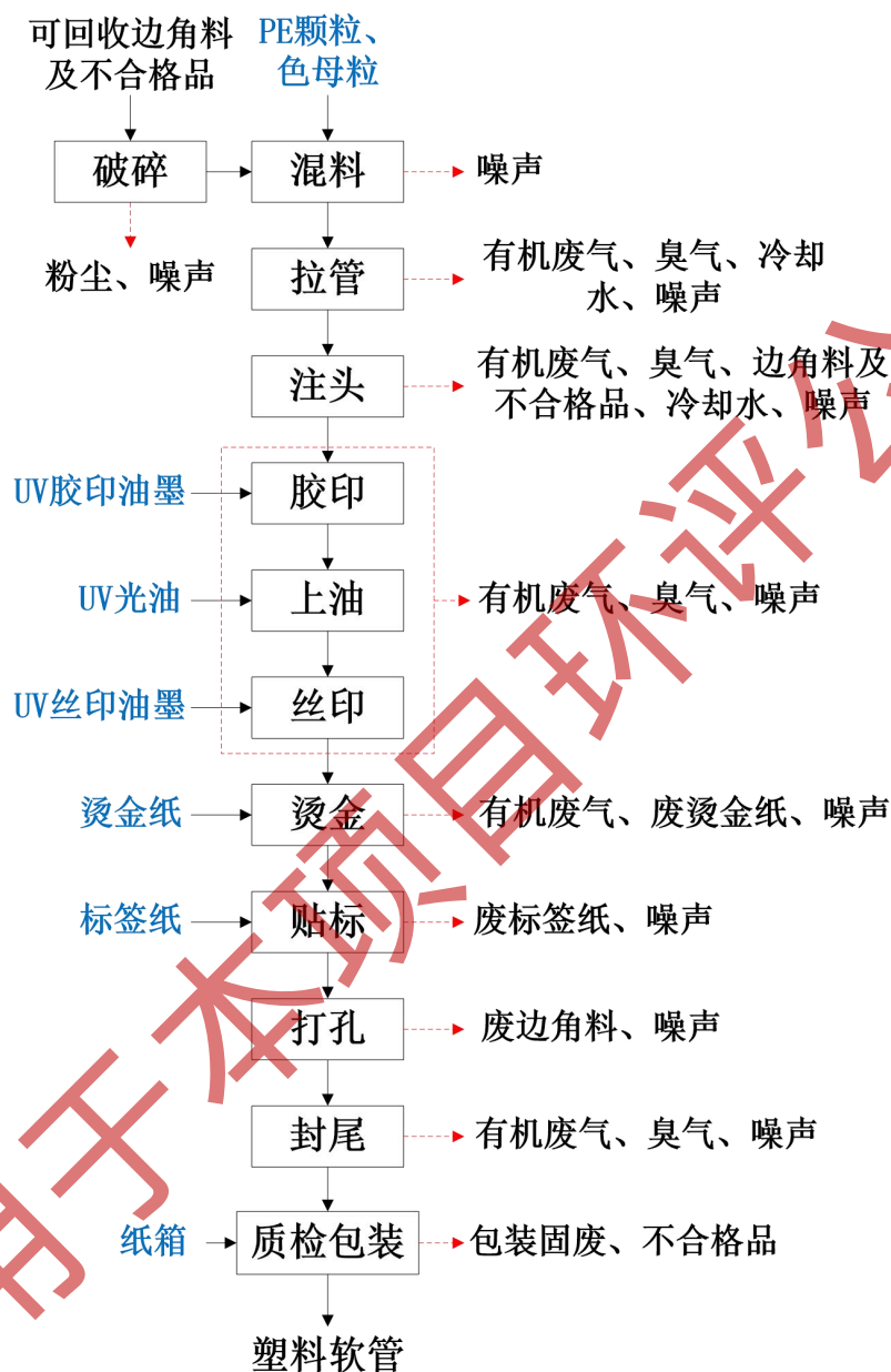
图 2-3 塑料软管生产工艺流程及产污节点图
