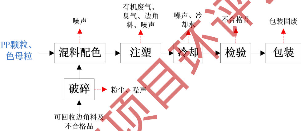
图 2-4 塑料盖生产工艺流程及产污节点图
