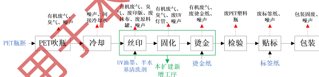
图 2-7 PET 塑料瓶生产工艺流程及产污节点图
