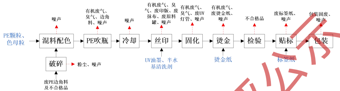
图 2-5 PE 塑料瓶生产工艺流程及产污节点图
