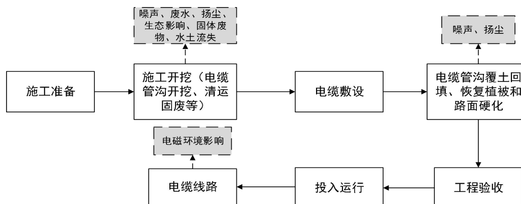
图 2-6 电缆沟施工工艺流程及产污环节图
