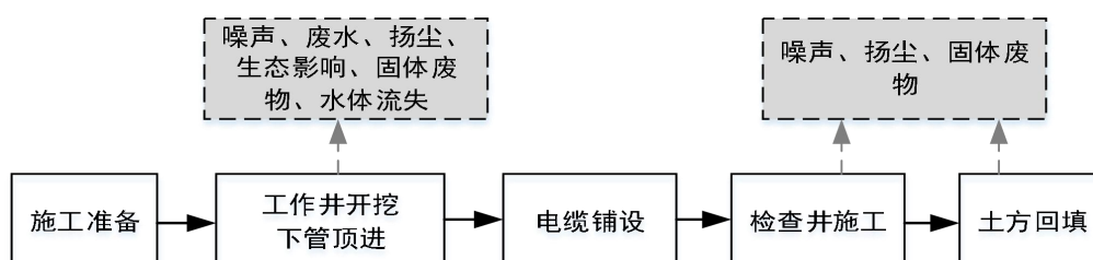
图 2-8 本项目电缆顶管施工工艺流程示意图
