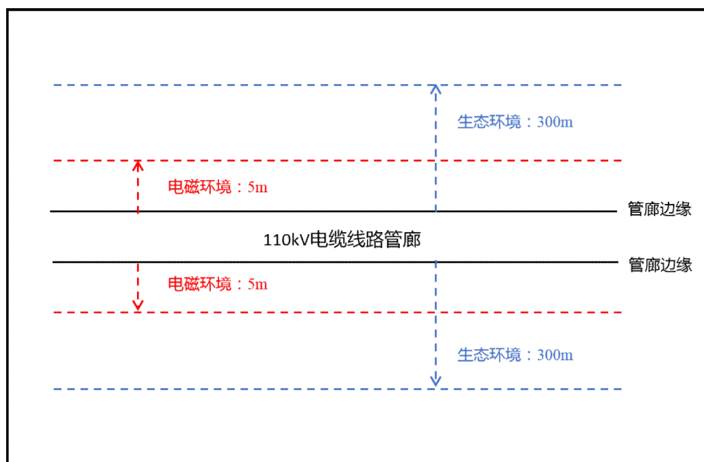
图 3-4 110kV 电缆线路评价范围示意图
