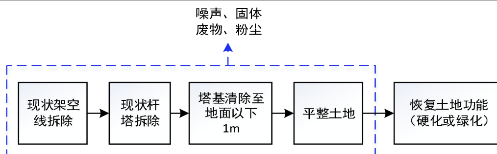
图 2-5 架空线路拆除工艺流程及产污环节图
