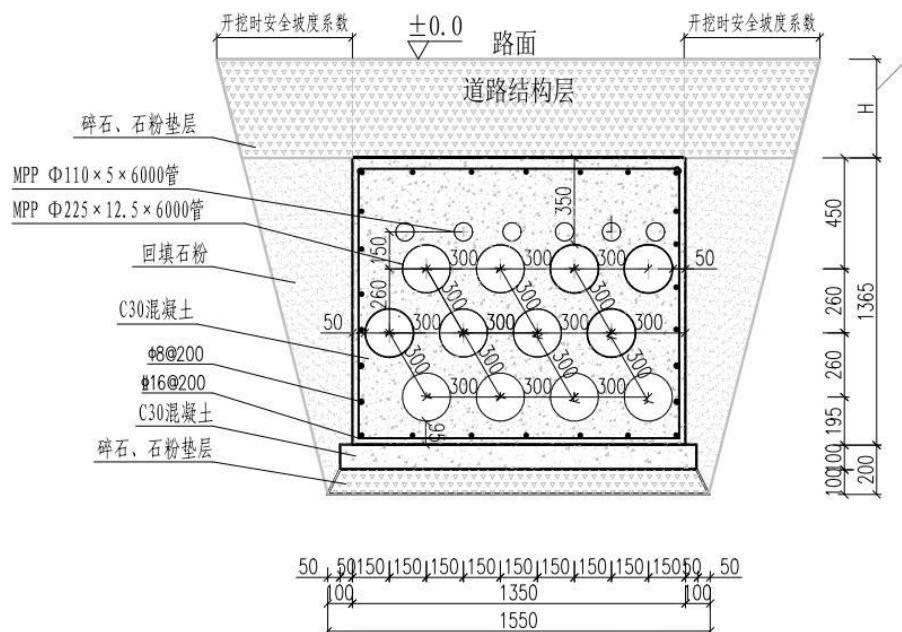
图 2-2 电缆埋管断面图
