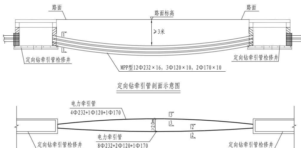
图 2-3 顶管示意图
