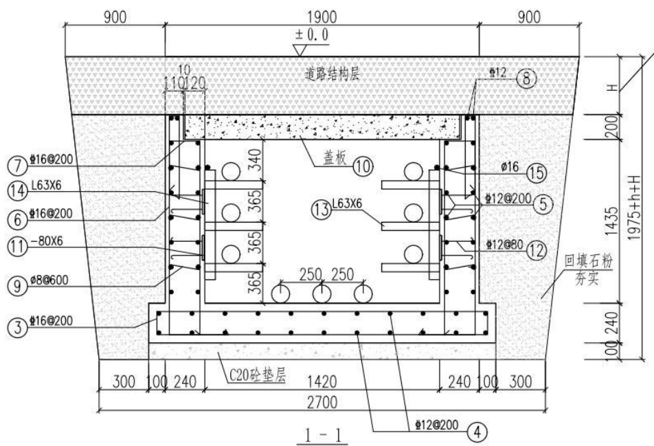
图 2-1 三回电缆沟断面图
