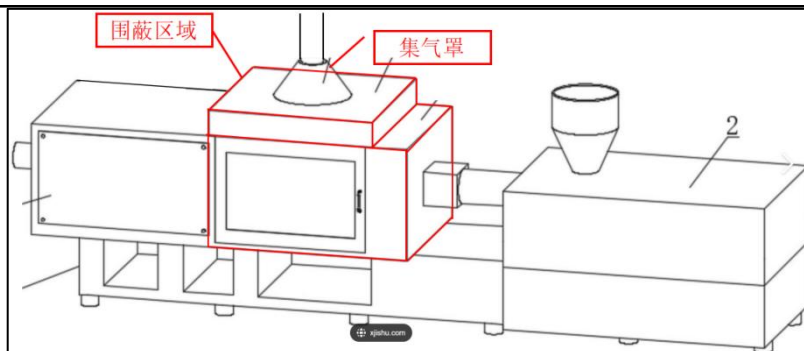
图 4-1 本项目注塑废气收集示意
