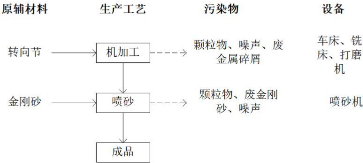
图 2-2 转向节的生产工艺流程
