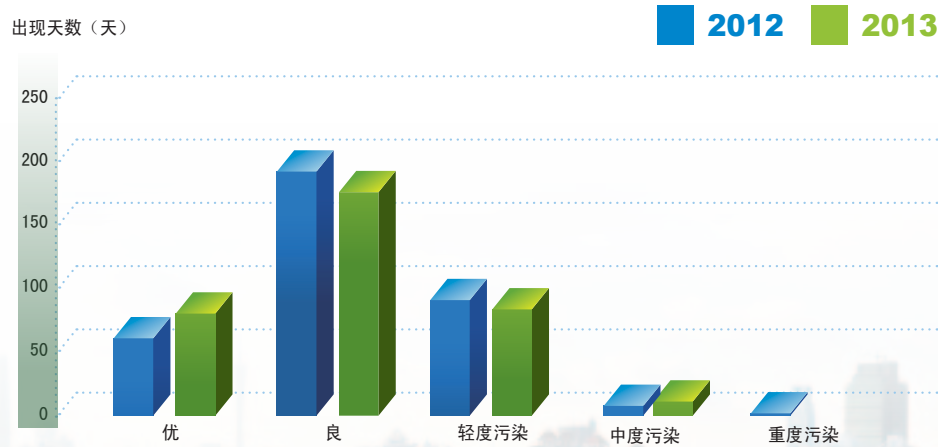
2013 年广州市环境空气质量状况
