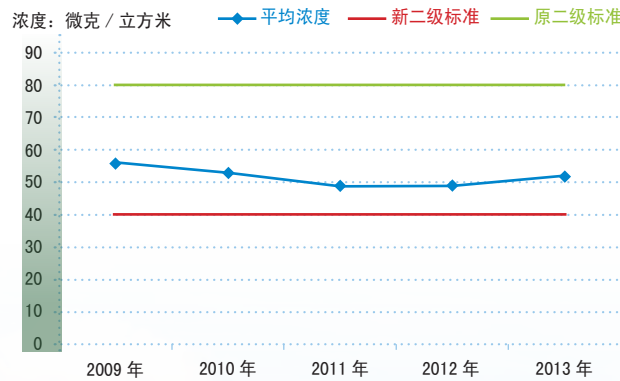
2009 ~ 2013 年广州市 NO 2 平均浓度变化趋势
