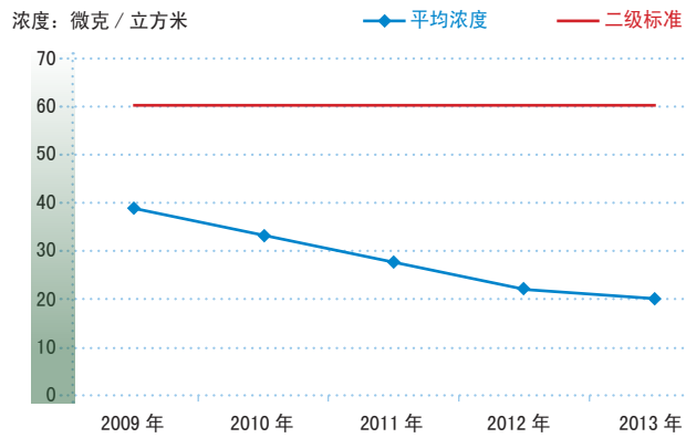
2009 ~ 2013 年广州市 SO 2 平均浓度变化趋势
