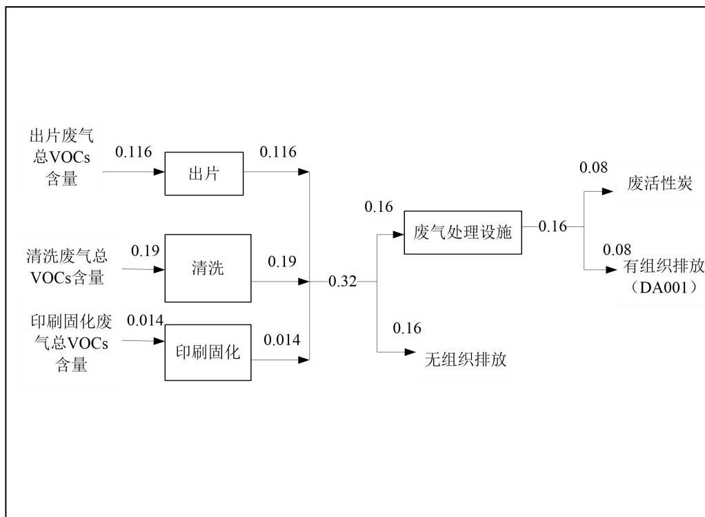
图 2-2 VOCs 平衡图
