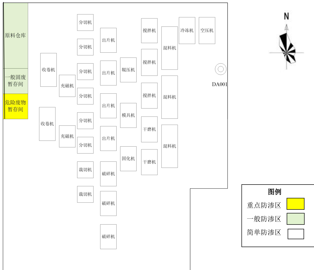
附图 2 厂区平面布置图及分区防渗图 (1 : 300)
