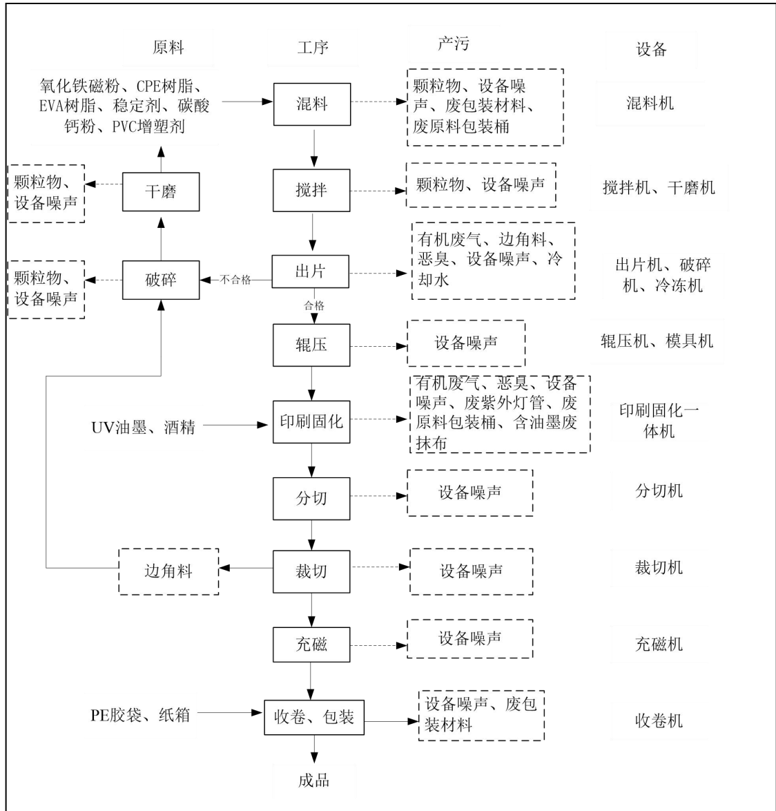
图 2-3 本项目生产工艺流程图
