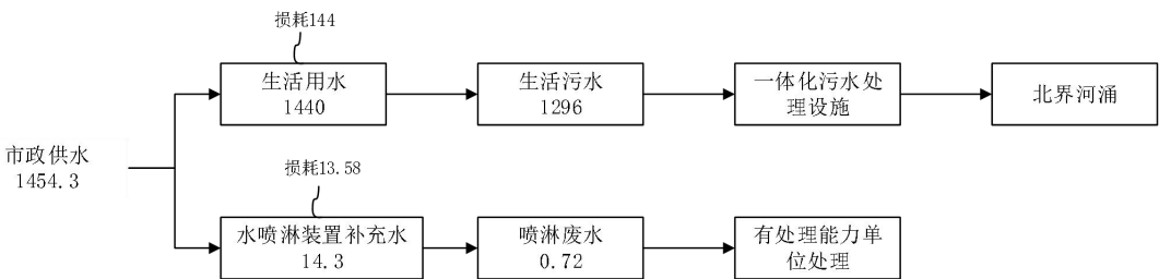
图 2-1 扩建后全厂水平衡图 单位 t/a
