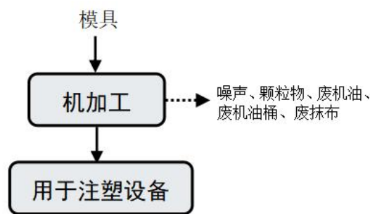
图 2-3 模具维修工艺流程及产污环节图
