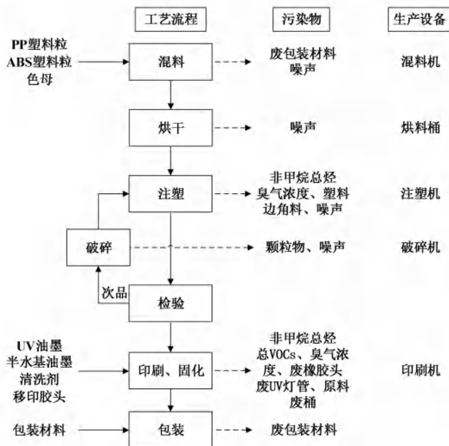
图 2-3 本项目音响塑料配件生产工艺流程及产污环节图
