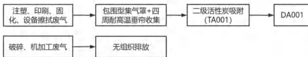
图 4-1 废气治理设施流程图
