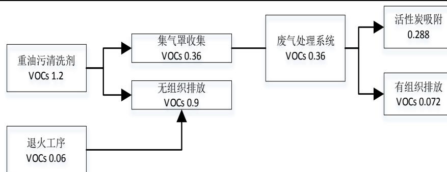
图 2-1 VOCs 平衡图（单位：t/a）
