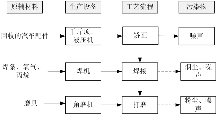
图 2-3 项目生产工艺流程及产污环节图
