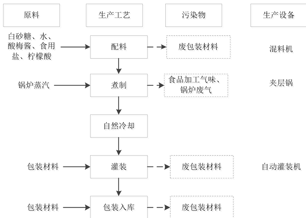
图 2-5 调味糖浆生产工艺流程图
