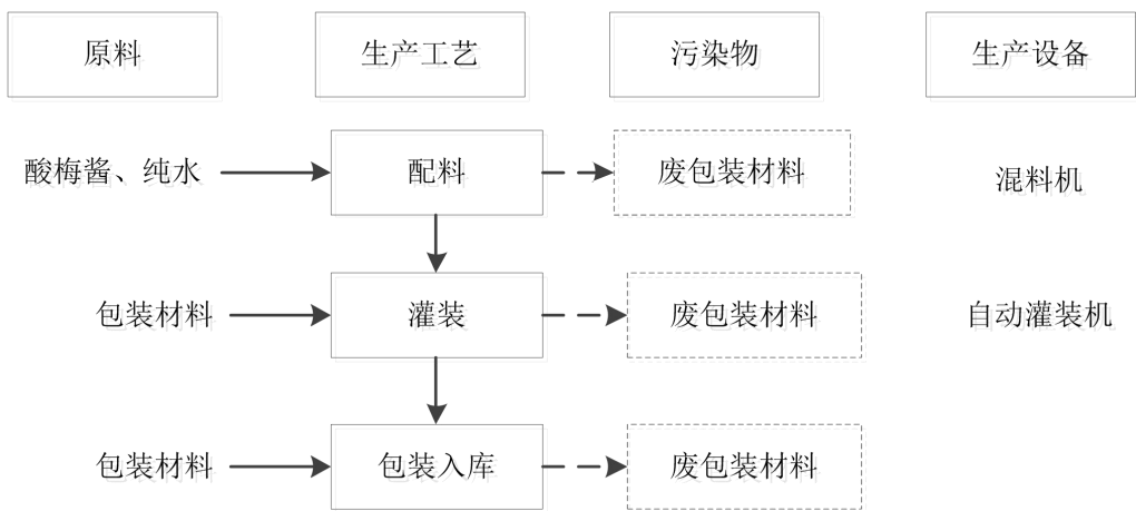
图 2-5 酸梅酱生产工艺流程图
