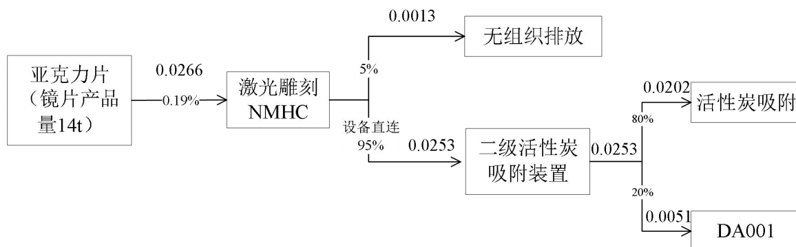
图 4-1 有机废气平衡图 单位:t/a
