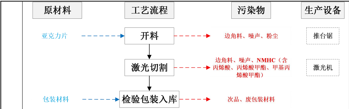
图 2-3 亚克力镜片生产工艺流程和产排污环节图
