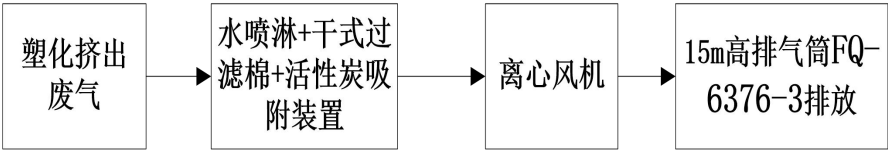
图 4-3 废气处理工艺流程图
